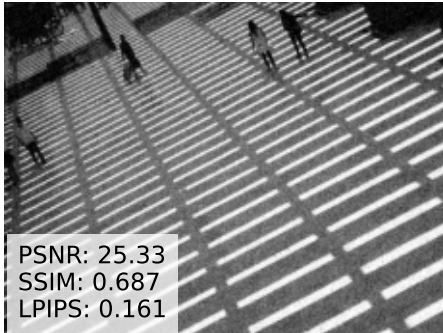
Noisy
