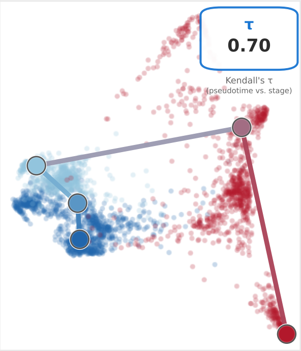
Diffusion Manifold
