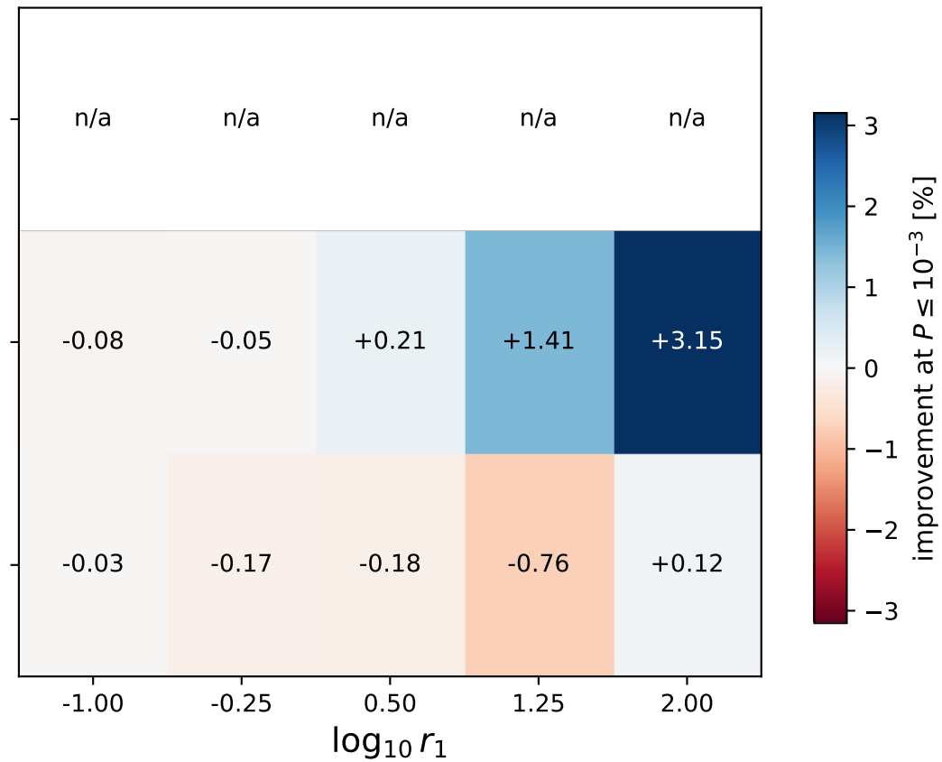
P1+P2 (protect)
