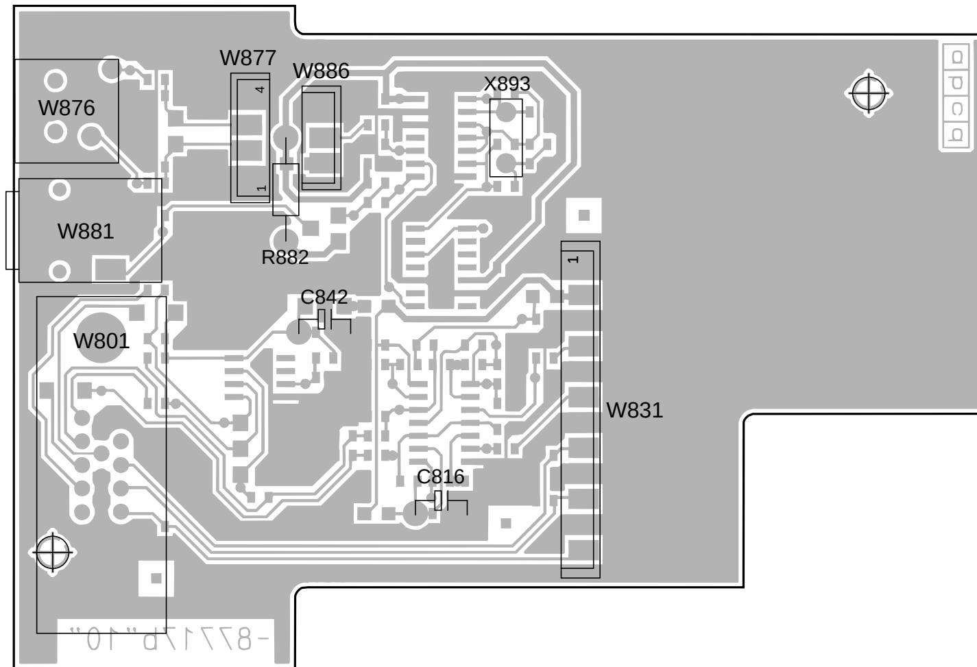
Ltpl. VGA IR Adapter 396-87717.050 Bestückungsseite - Components side
