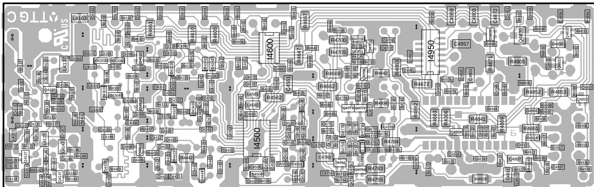
LtpI. Tuner/ZF Tuner/IF P.C.B Bestückungsseite • Components side
