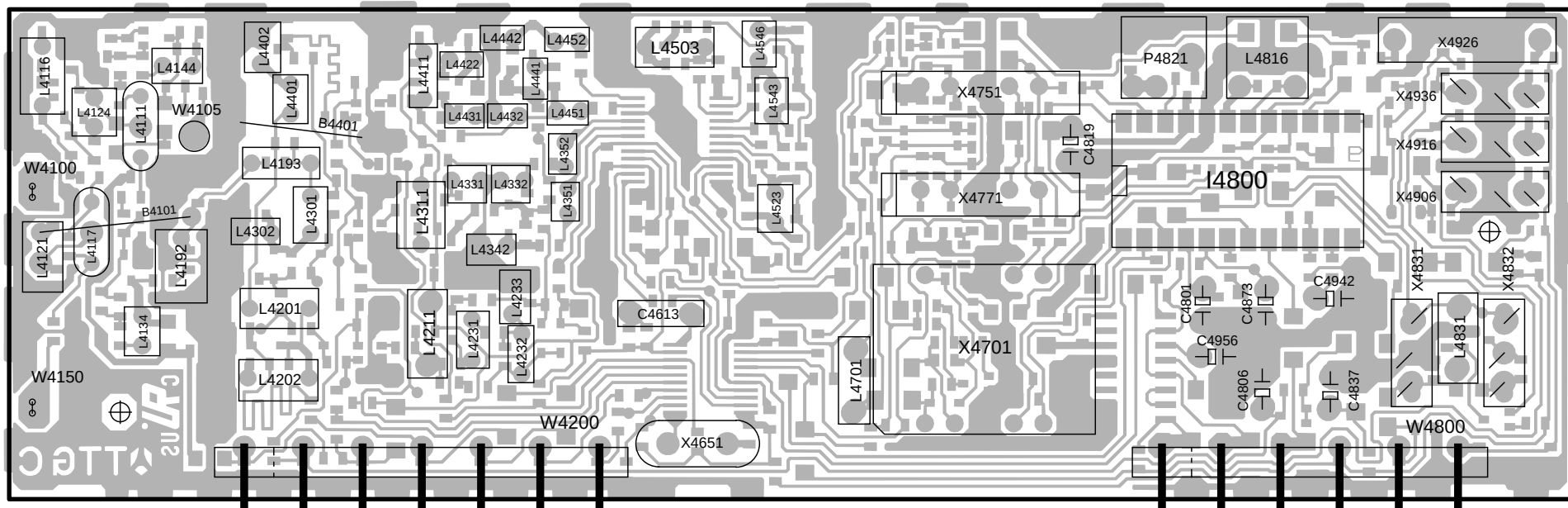
LtpI. Tuner/ZF Tuner/IF P.C.B Bestückungsseite • Components side
