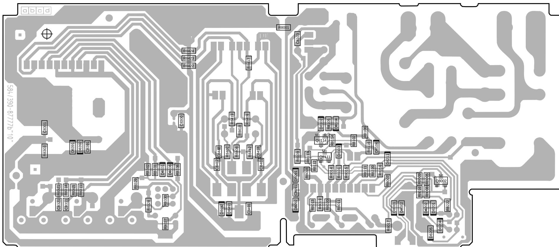
LtpI. Bedienteil Control Board Lötseite • Solder side
