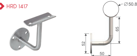
SOPORTE BARANDAL A MURO.
