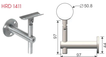
SOPORTE BARANDAL AJUSTABLE MURO - TUBO.
