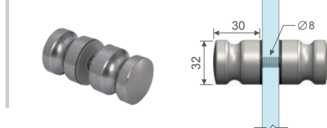
POMO CONECTOR PARA VIDRIOS.
