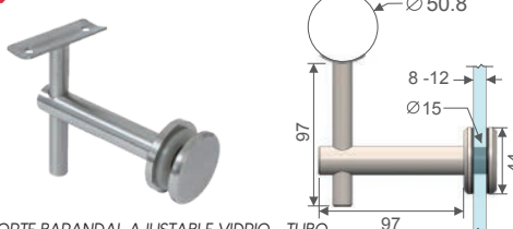
SOPORTE BARANDAL AJUSTABLE VIDRIO - TUBO.
