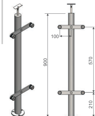
➤ HRD 1520 ➤ HRD 1522 NEGRO
