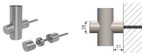
CONECTOR PARA TUBO BARANDAL CACHETEADO.
