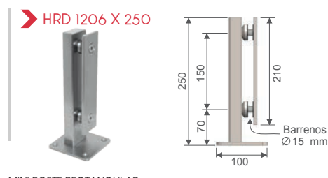
MINI POSTE RECTANGULAR
