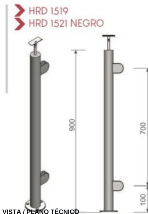
VISTA / PLANO TÉCNICO
