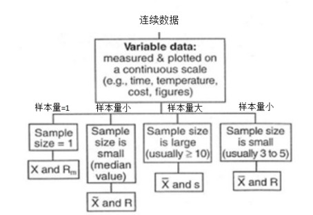
基于样本多少选择恰当的控制图
