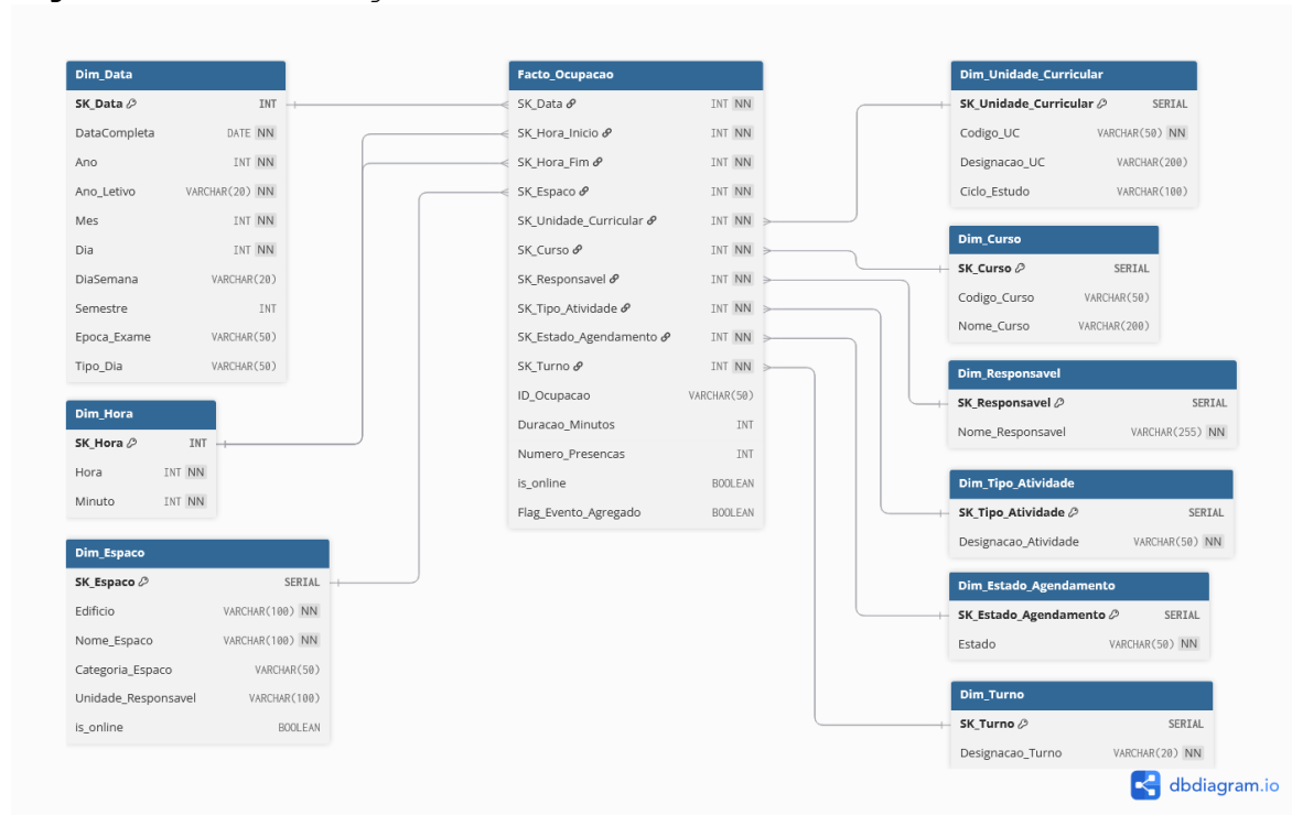
Figura 2.2 – Diagrama do Modelo Dimensional ESTG Star Schema.
