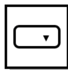
DROPDOWN
