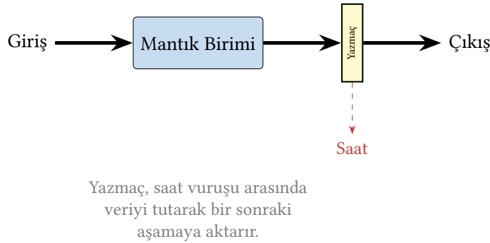
Şekil 6.18: Mantık birimine ara yazmaç konulması
