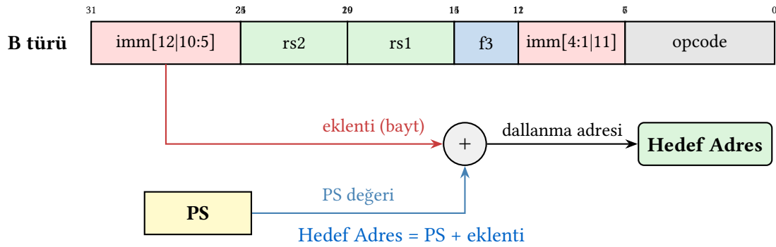
Şekil 3.17: RISC-V'te PS'ye Göreceli Adresleme Kipi
