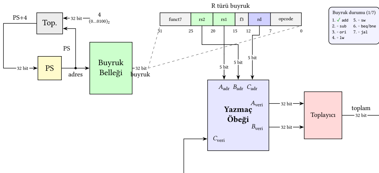
Şekil 6.3: add buyruğunu yürütebilen yalın veri yolu. Yazmaç öbeğinin üç adres girişi vardır: A_{\text{adr}} ve B_{\text{adr}} okunacak iki yazarın numarasını, C_{\text{adr}} ise sonucun yazılacağı yazarın numarasını alır. Buyruktan çıkan rs1 ve rs2 alanları A_{\text{adr}} ve B_{\text{adr}} 'a, rd alanı C_{\text{adr}} 'a bağlanır. Karşılığında veri çıkışları A_{\text{veri}} ve B_{\text{veri}} toplayıcıya, toplayıcı sonucu da C_{\text{veri}} üzerinden yazmaç öbeğine geri yazılır. PS ayrı bir toplayıcıyla 4 artırılır. Bu basit veri yolunda henüz hiçbir denetim sinyali yoktur: bütün yollar her saat çevriminde aktiftir.
