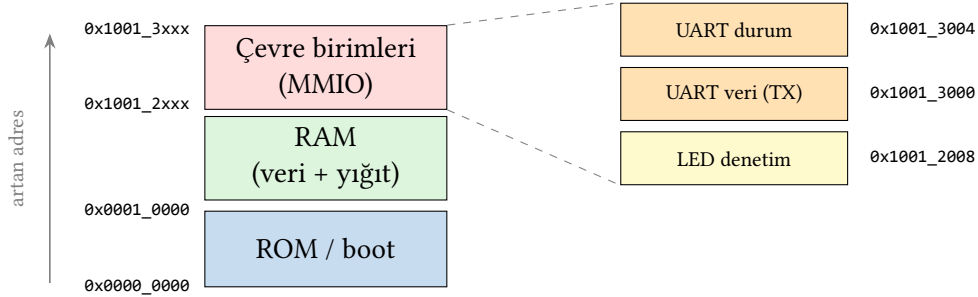
Şekil 4.15: Gömülü sistemde bellek eşlemeli giriş/çıkış adres haritası. Adres uzayının alt bölgeleri ROM ve RAM'e, üst bölgesi çevre birimlerine ayrılmıştır. Sağdaki yakınlaştırma, çevre birim bölgesindeki UART ve LED yazmaçlarını gerçek adresleriyle gösterir. Bu adreslere 1w/sw ile erişmek doğrudan donanımı sürer.
