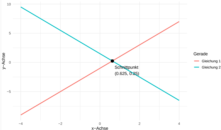
Graph der beiden Geraden mit Schnittpunkt
