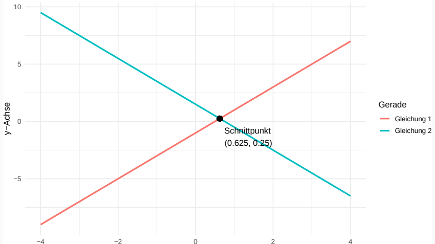
Graph der beiden Geraden mit Schnittpunkt
