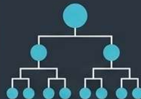
Diagramma Gerarchico
