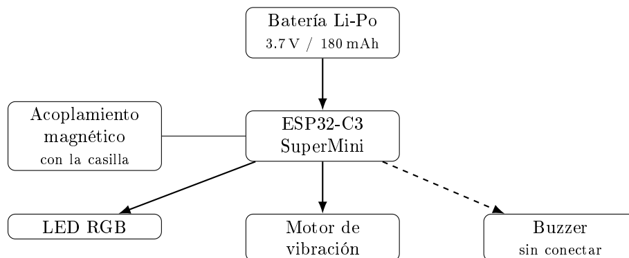
Figure 4.6: Arquitectura interna del cubo inteligente: un microcontrolador ESP32-C3 SuperMini gestiona dos actuadores multisensoriales (LED RGB y motor de vibración) y se alimenta de una batería Li-Po. La placa incluye además un buzzer (trazo discontinuo) sin conexión eléctrica activa al microcontrolador, por lo que no forma parte de la respuesta multisensorial del sistema — el sonido lo emite en su lugar el computador del docente, como se explica en el texto. El trazo delgado hacia el acoplamiento magnético señala una relación mecánica de posicionamiento con la casilla de la base, distinta de las señales de control eléctricas que el microcontrolador gestiona directamente sobre el LED y el motor de vibración.
