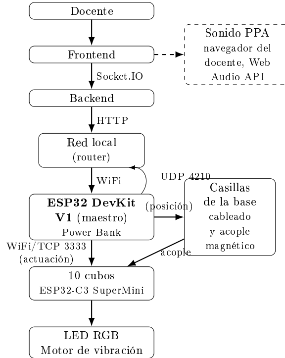
Figure 4.7: Arquitectura general del sistema. El ESP32 DevKit V1 (maestro) se conecta a la red local del laboratorio a través de un router y sostiene, hacia los diez cubos, dos canales independientes: uno de actuación (WiFi, mediante una conexión TCP en el puerto 3333), por el que transmite los comandos de color y vibración, y uno de posición (cableado de las casillas de la base y su acoplamiento magnético con cada cubo), por el que detecta en qué posición del tablero se encuentra cada uno. El sonido de cada fase del PPA no viaja por ninguno de estos dos canales (recuadro discontinuo): lo emite directamente el navegador del docente mediante la API de audio del navegador (Web Audio API), en sincronía con la orden enviada al cubo.
