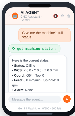
AI agent · function calling (Gemini)
