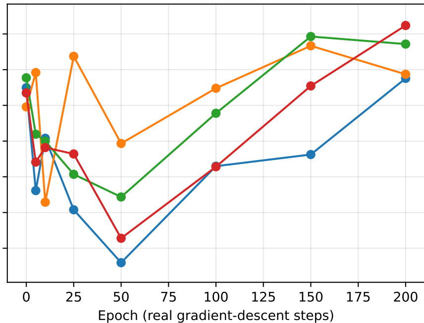
cifar
