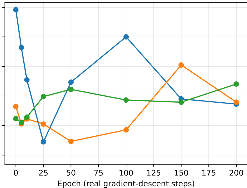
cifar
