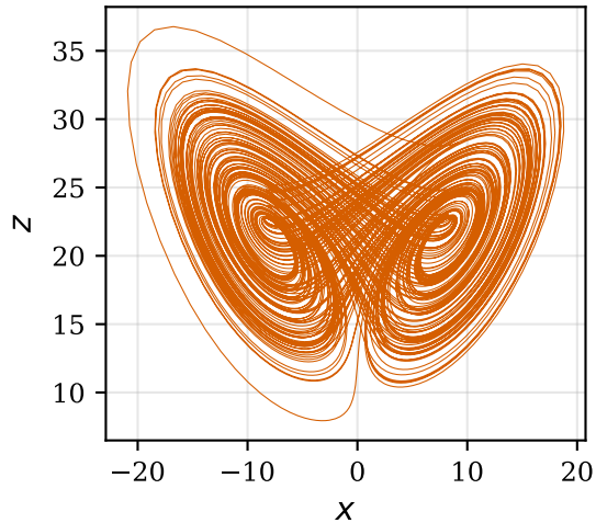
(b) x - z
