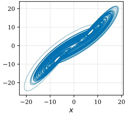
(a) x - y
