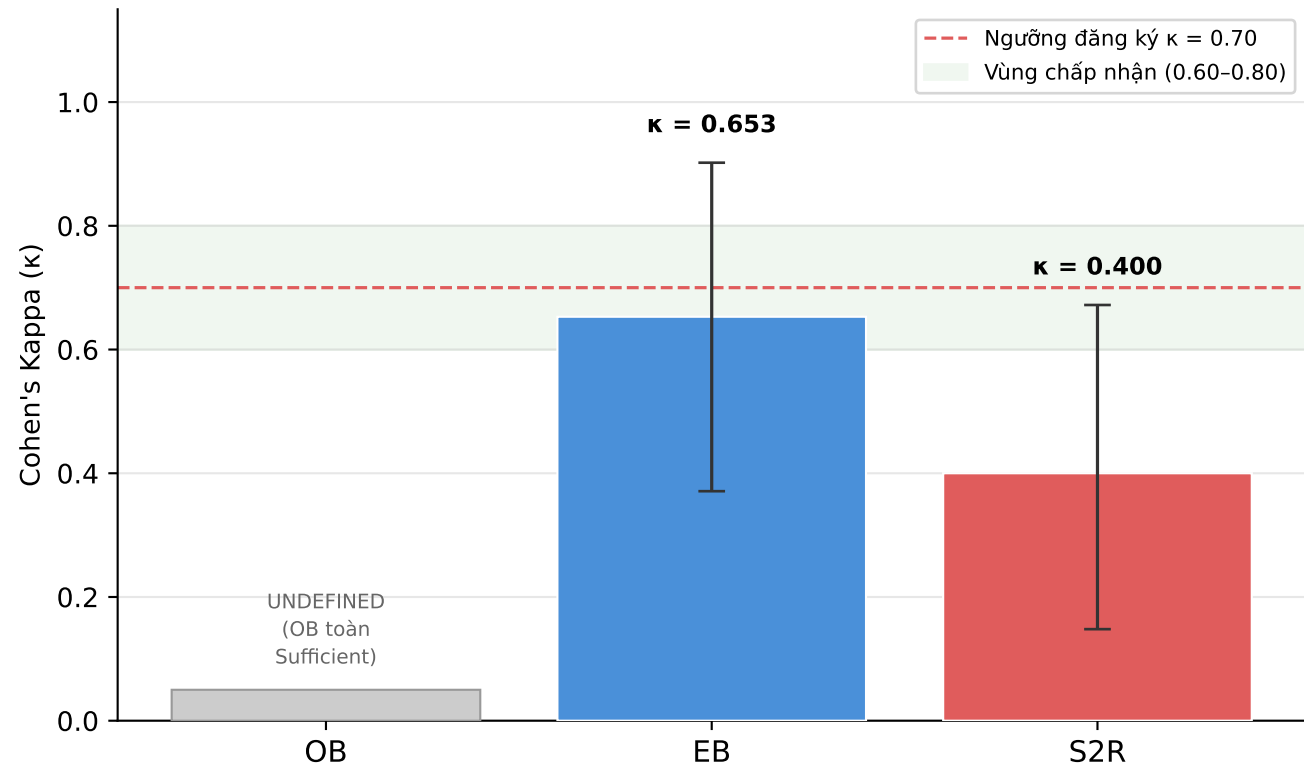
Kappa LLM-vs-Developer theo từng component (pilot, N=30)
