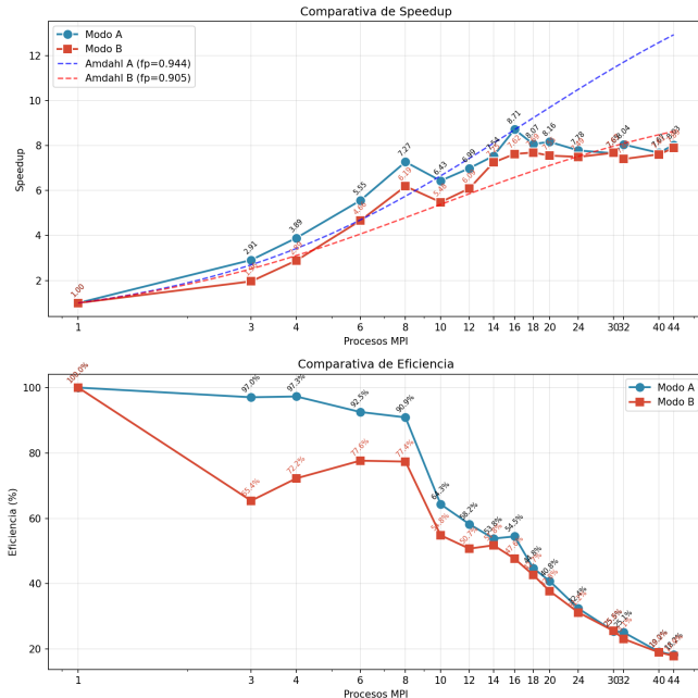
Figura 6: Comparativa de speedup entre Modo A y Modo B. El Modo A supera al Modo B en todos los rangos, alcanzando un speedup máximo de 8.71x con 16 procesos.
