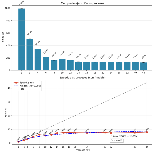
Figura 5: Speedup real, curva de Amdahl ( f_p = 0,905 ) e ideal (en Modo B).
