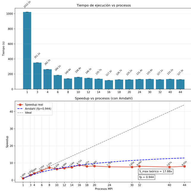
Figura 4: Speedup real, curva de Amdahl ( f_p = 0,944 ) e ideal (en el denominado Modo A de los ensayos).
