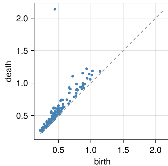
H 1 — Lorenz
