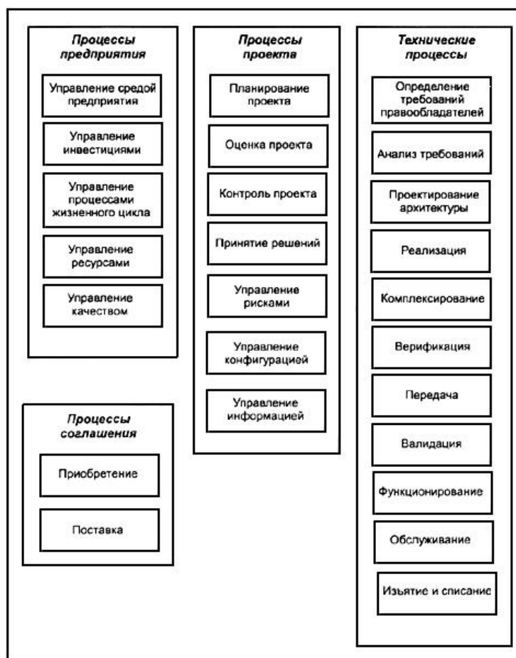
Рисунок D.8 - Процессы жизненного цикла системы
