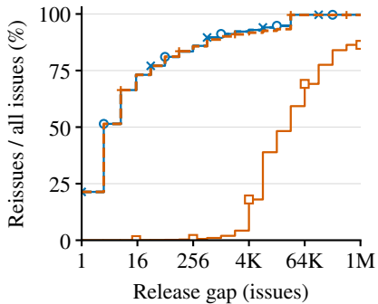
(a) Same-start reuse
