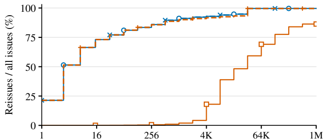
(a) SQLite · memsys5 speedtest1 main
