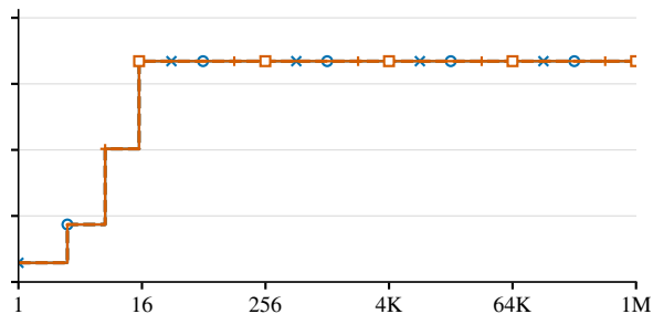
(d) FFmpeg · pool leases FATE Xvid, 20 frames
