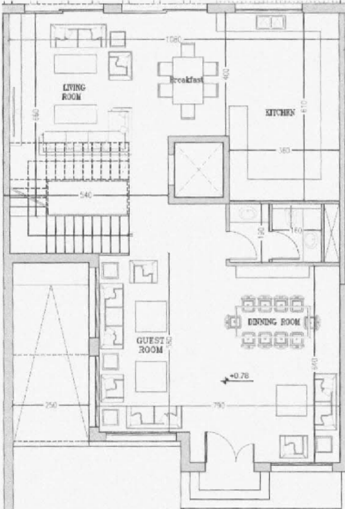
مخطط هندسي للطابق الأرضي (VILLA (C))
