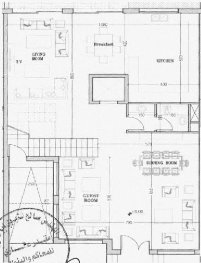
مخطط هندسي للطابق الأرضي (VILLA (B))
