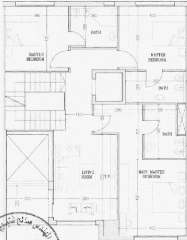
مخطط هندسي للطابق الأول (VILLA (C))
