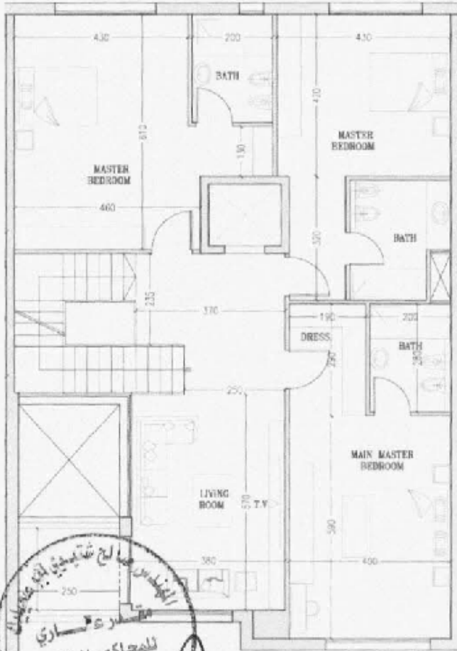
مخطط هندسي للطابق الأول (VILLA (B))
