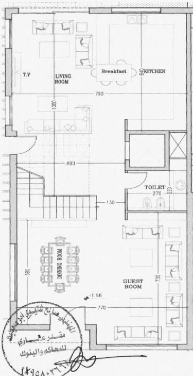
مخطط هندسي للطابق الأرضي (VILLA (A))
