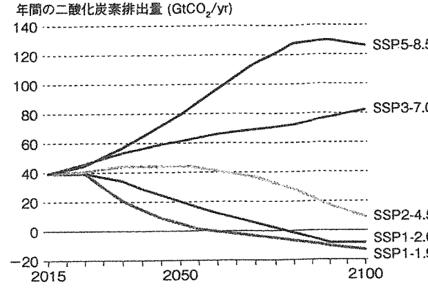
図2 図1のSSPに対応する世界の二酸化炭素排出量。(出典：IPCC AR6 SPMを元に作成)
