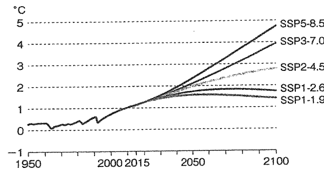
図1 1850～1900年を基準とした世界平均気温の変化。今世紀末の温暖化は、最小では1.5℃程度、最大では5℃程度と予想されている。この変化をもたらすのは、我々人類の選択だ (出典：IPCC AR6 SPMを元に作成)
