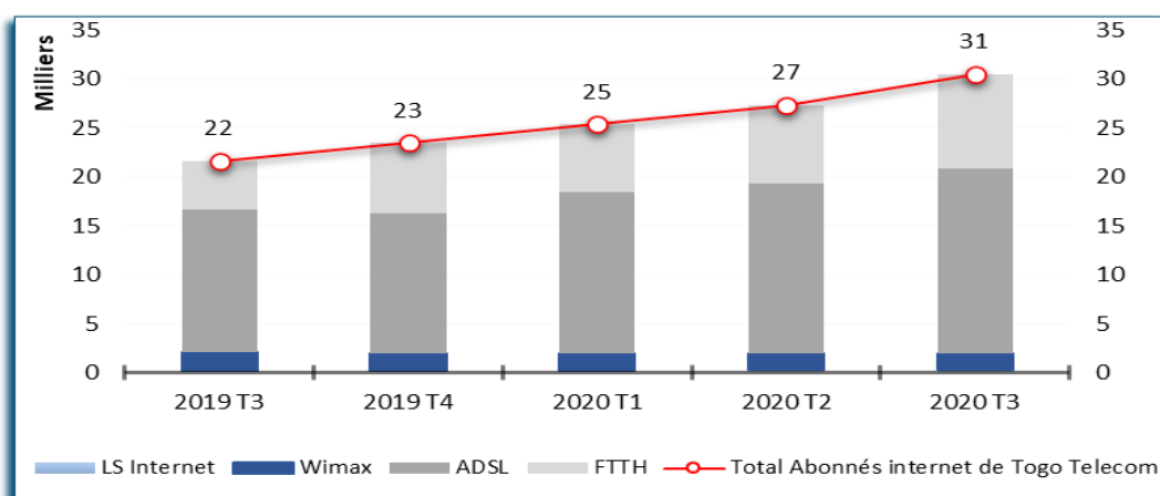
Graphique 10 : Evolution du nombre d'abonnés Internet de Togo Telecom par type d'accès
