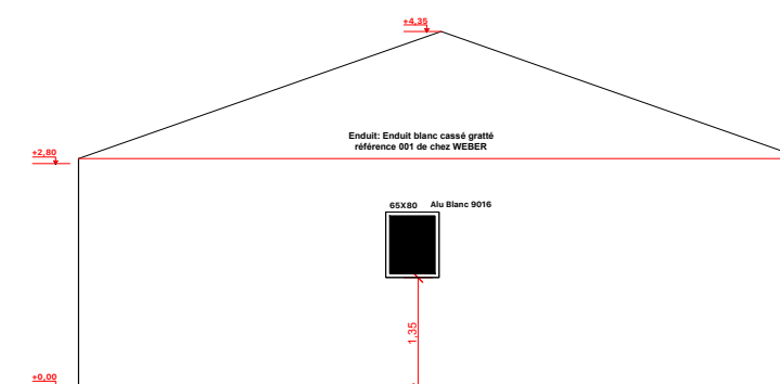
Façade Est
