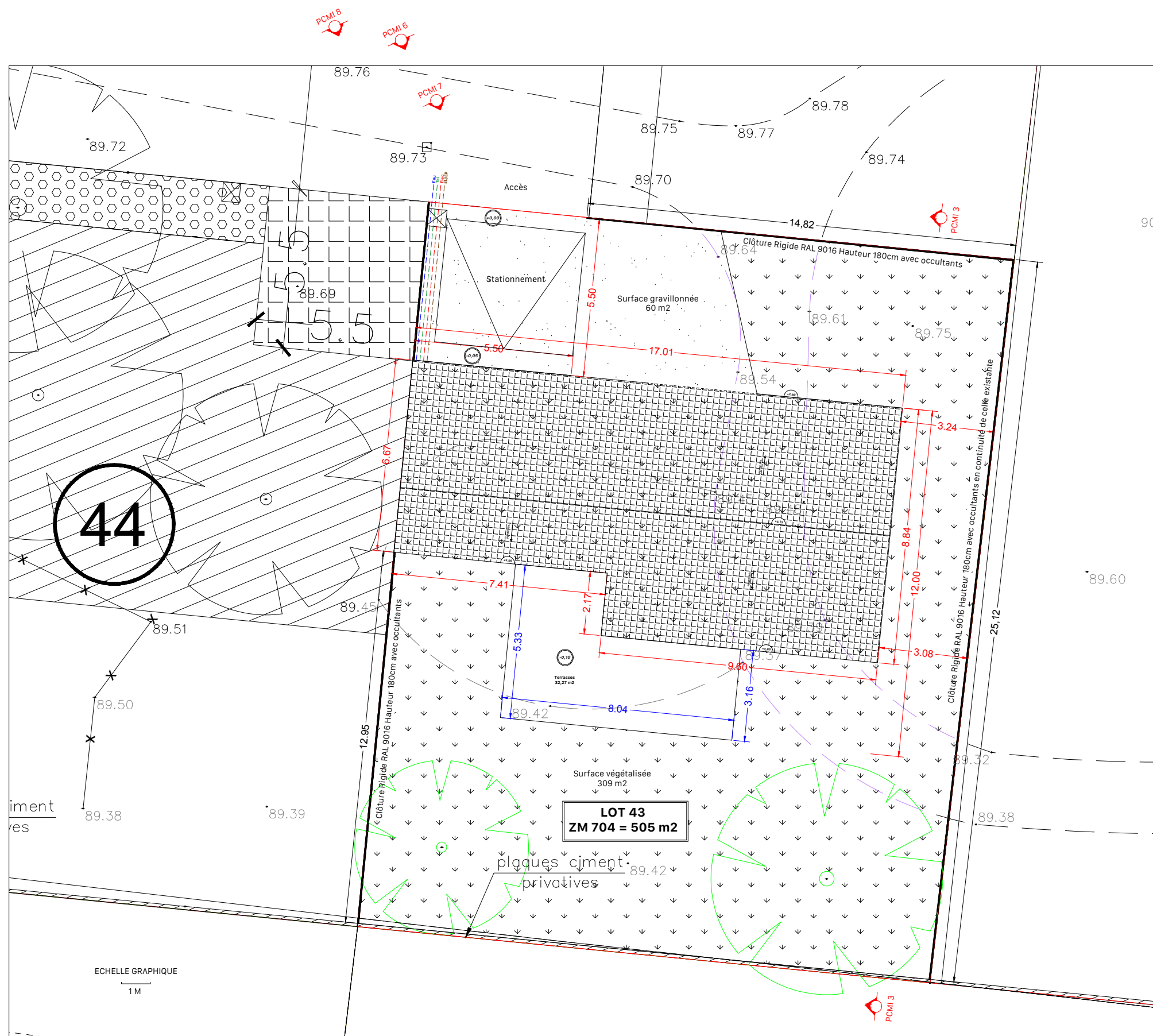
PCMI 2 - Plan de masse Projeté
