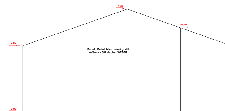
Façade Ouest
