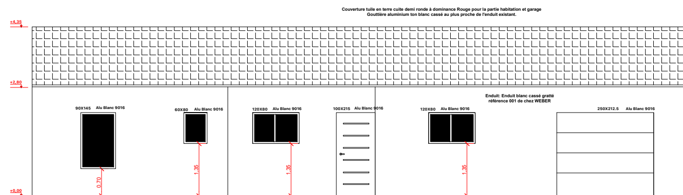
Façade Nord
