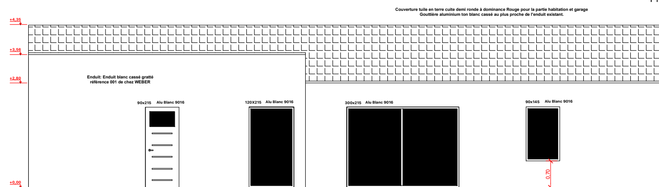
Façade Sud
