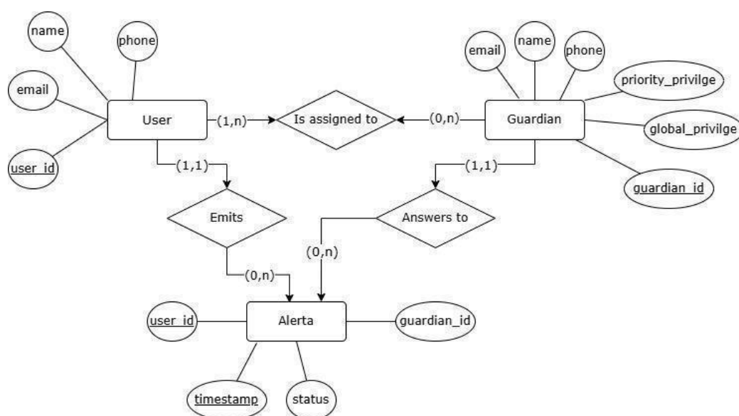
Diagrama 1 – Diagrama de entidade e relacionamento
