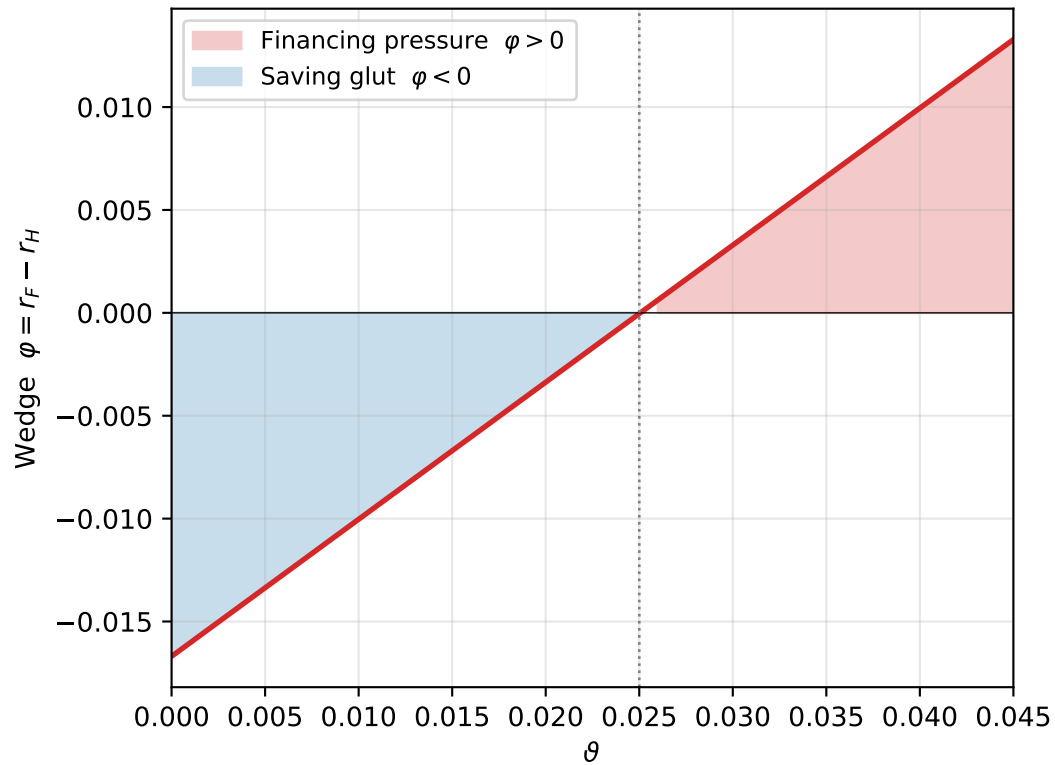
Phase 2(d) wedge
