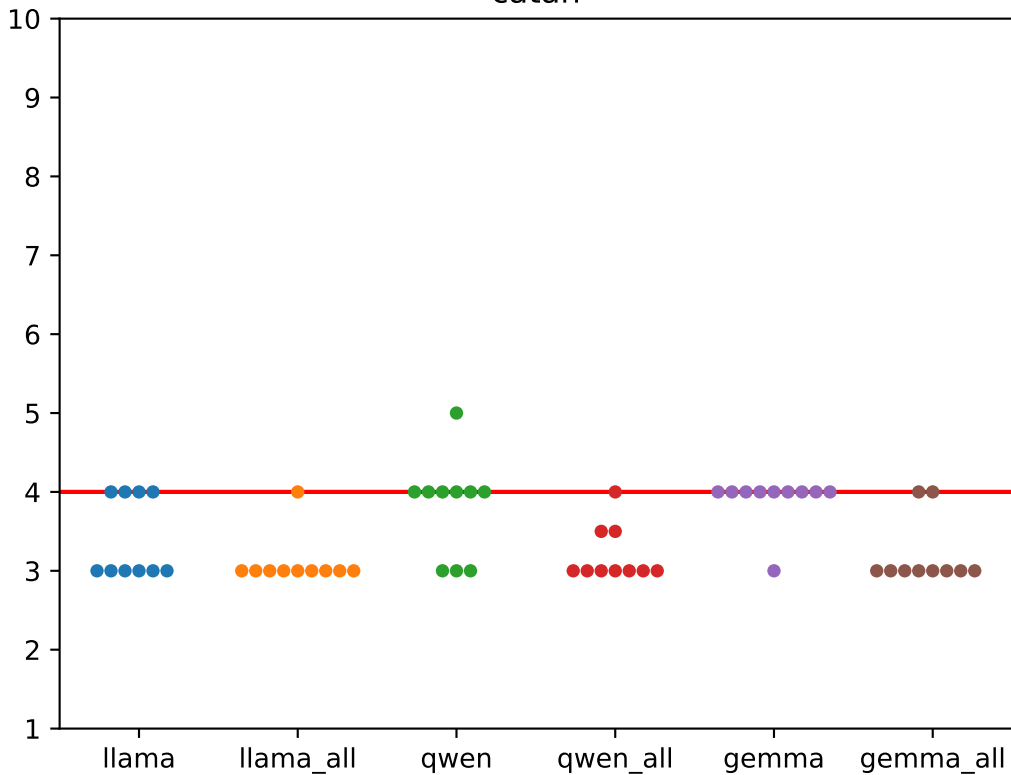
catan
