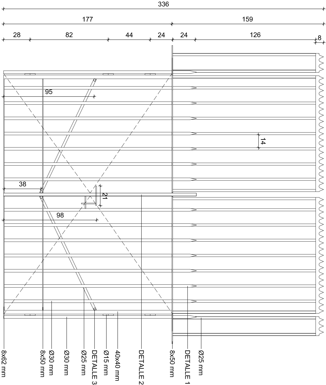
ELEVACIÓN Esc. 1/20
