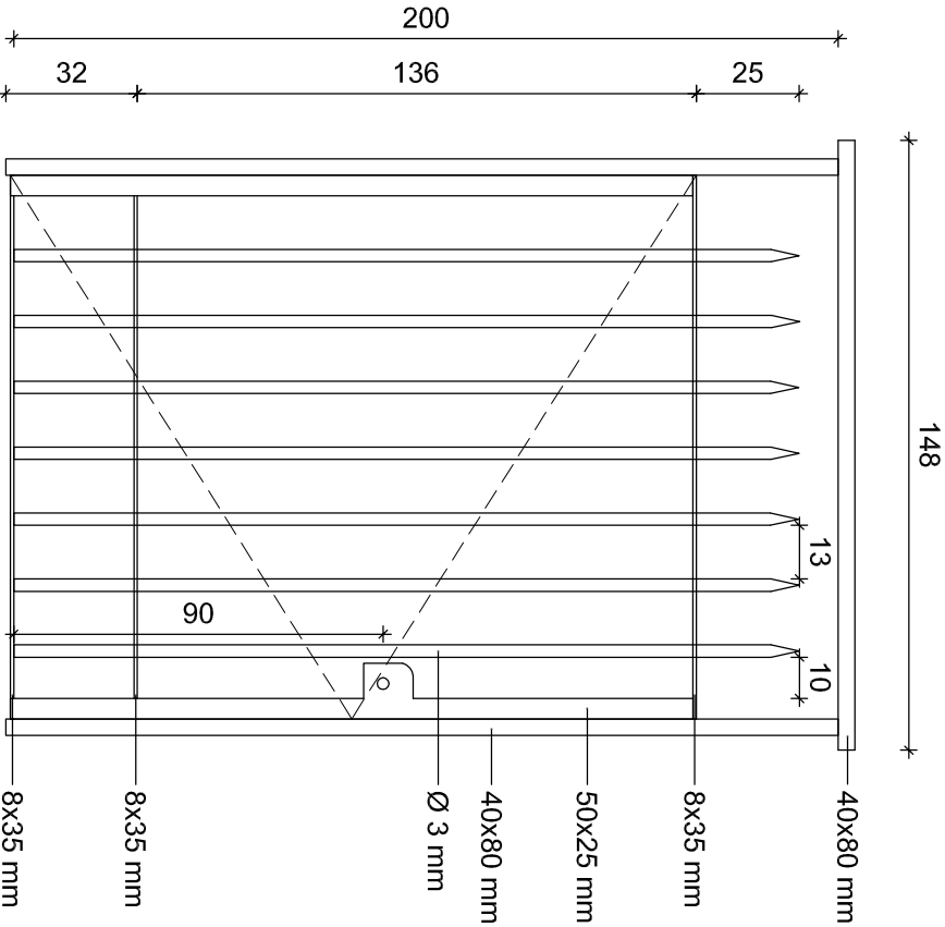
ELEVACIÓN Y PLANTA Re 05 y 08 Esc. 1/20
