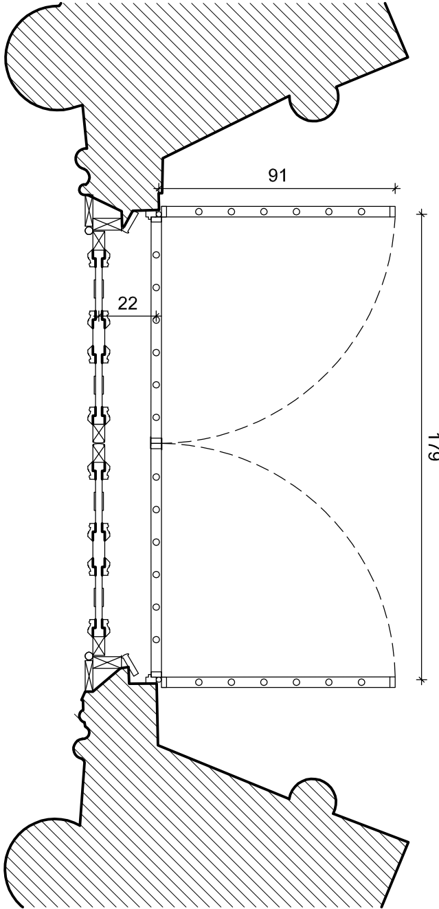
PLANTA Esc. 1/20
