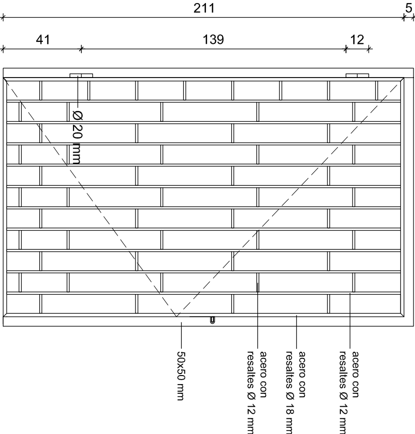
ELEVACIÓN Y PLANTA Re 03 y 04 Esc. 1/20
