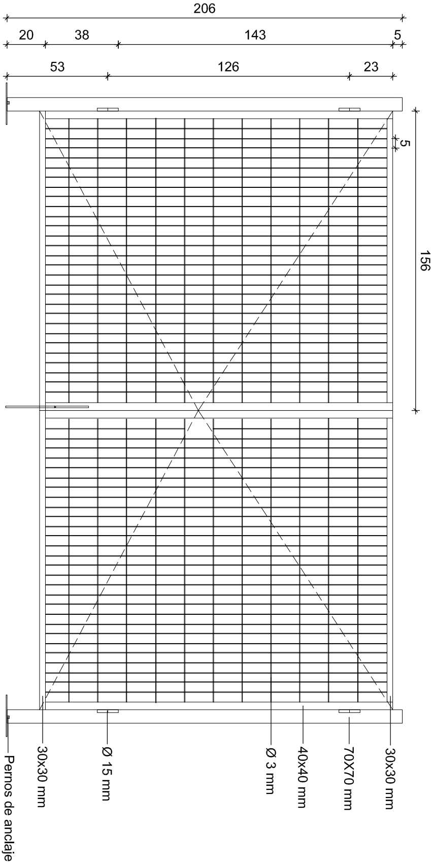
ELEVACIÓN PORTÓN ACCESO AGUSTINAS Esc. 1/20
