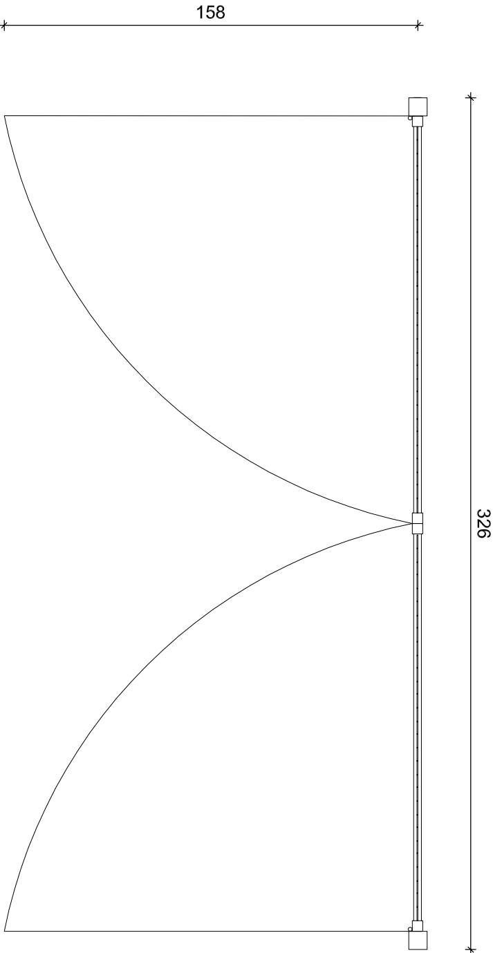
ELEVACIÓN PORTÓN ACCESO AGUSTINAS Esc. 1/20
