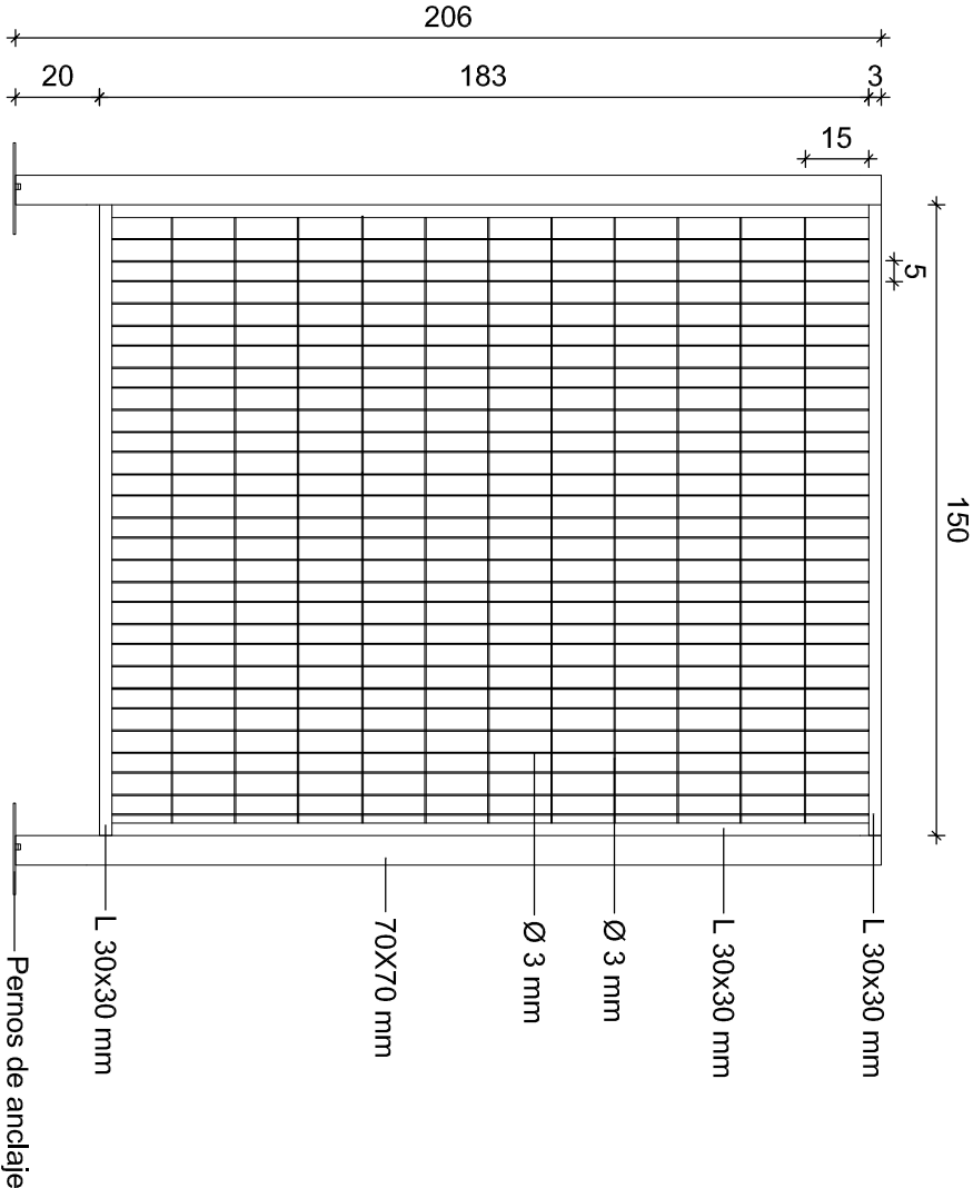
ELEVACIÓN MÓDULO TIPO REJA CALLE AGUSTINAS Y A. BARROSO Esc. 1/20
