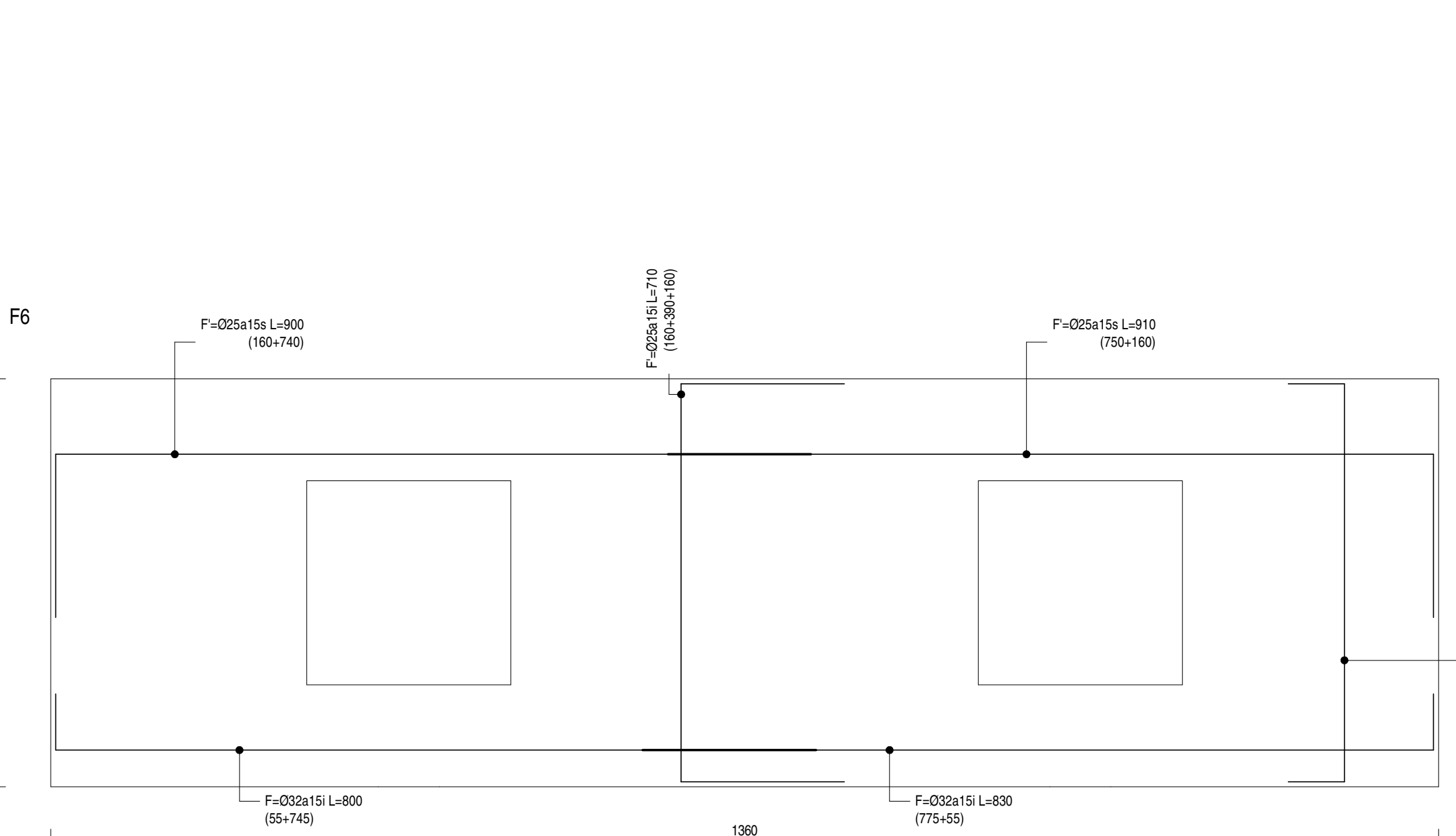
DETALLE TIPICO ARMADURA ZAPATA F6 ESCALA 1 : 50
