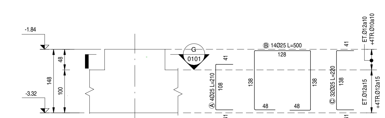
DETALLE TIPICO ARMADURA PEDESTAL PD2 ESCALA 1 : 50
