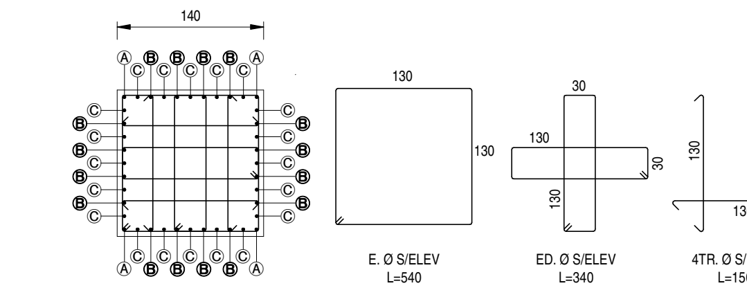
CORTE ESC. 1 : 50
