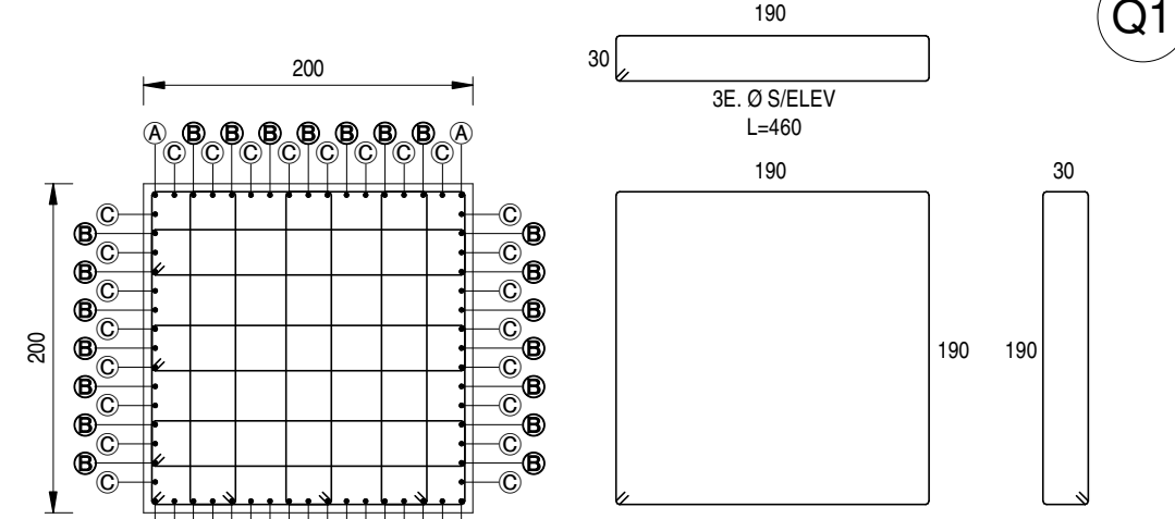
CORTE ESC. 1 : 50
