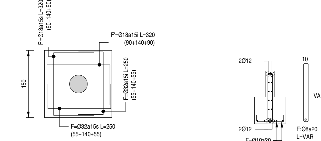
DETALLE TIPICO ARMADURA ZAPATA F8 ESCALA 1 : 50
