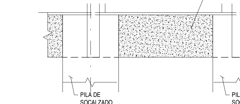
DETALLE TIPICO MURO DE CONTENCIÓN ENTRE PILAS ESCALA 1 : 50
