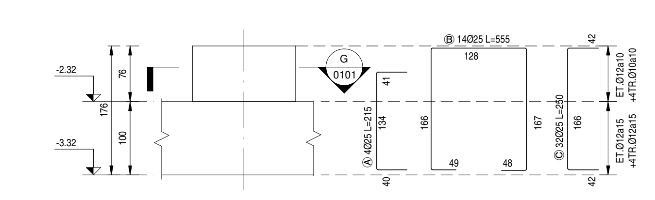
DETALLE TIPICO ARMADURA PEDESTAL PD3 ESCALA 1 : 50
