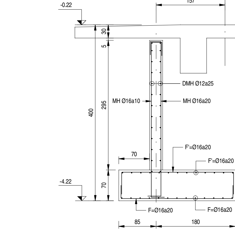
CORTE ESC. 1 : 50
