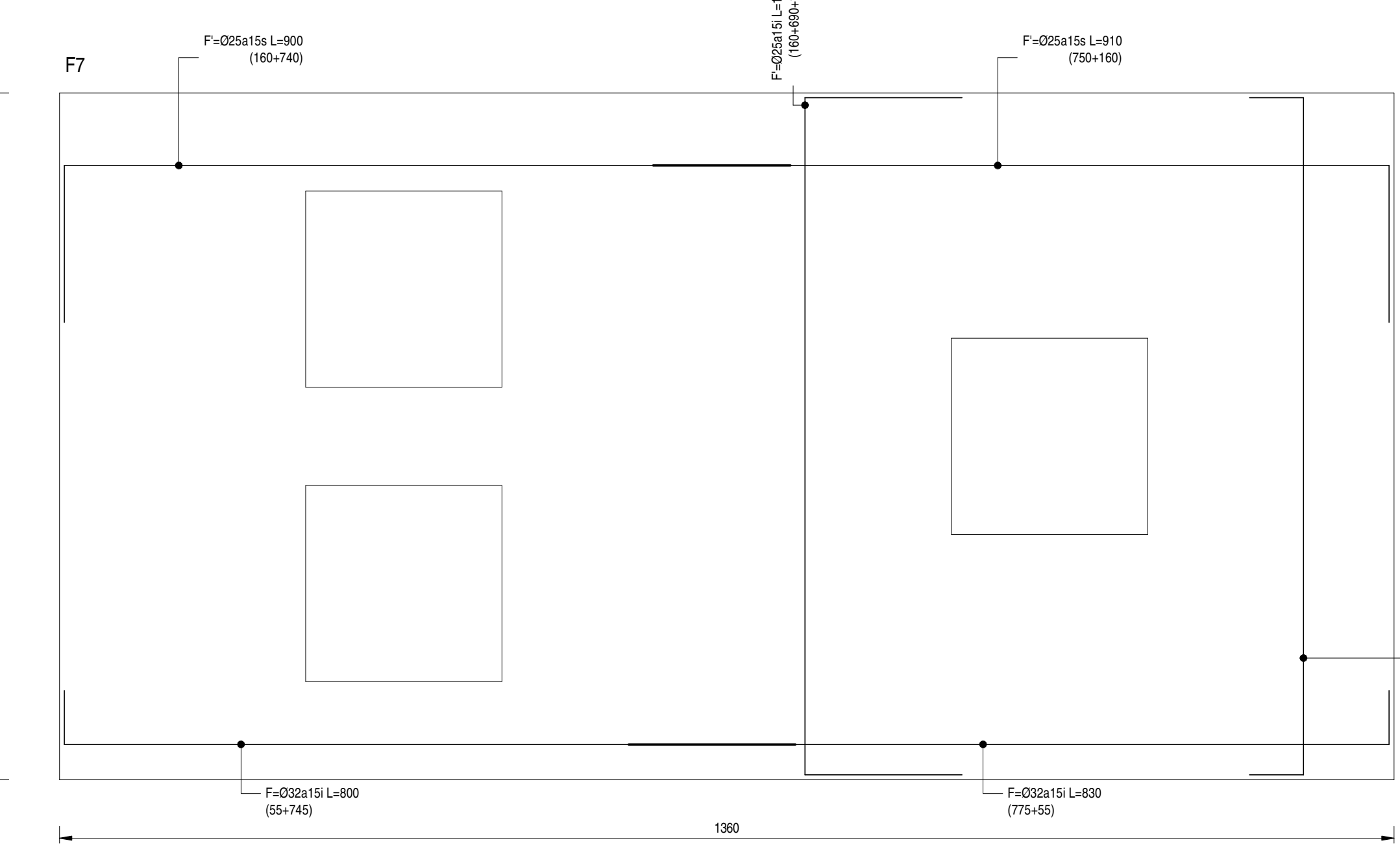
DETALLE TIPICO ARMADURA ZAPATA F7 ESCALA 1 : 50
