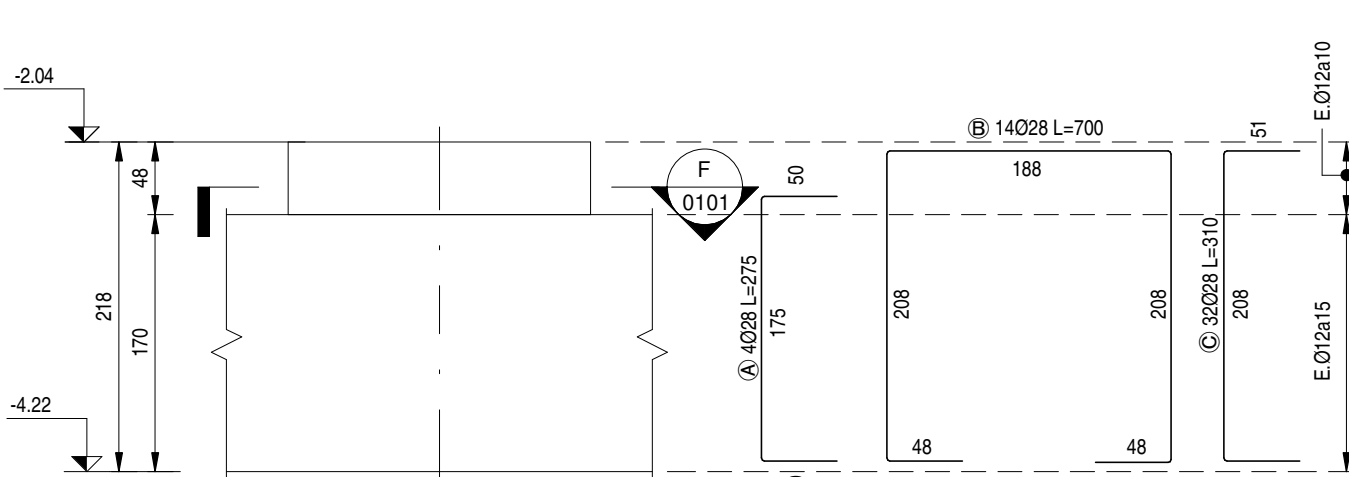
DETALLE TIPICO ARMADURA PEDESTAL PD1 ESCALA 1 : 50
