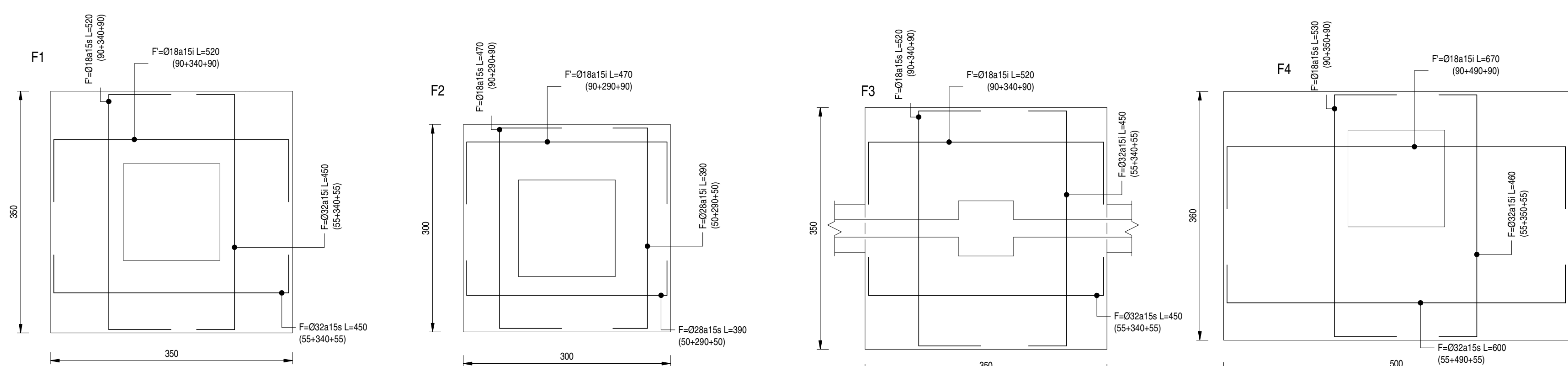
DETALLE TIPICO ARMADURA ZAPATA F1 ESCALA 1 : 50
