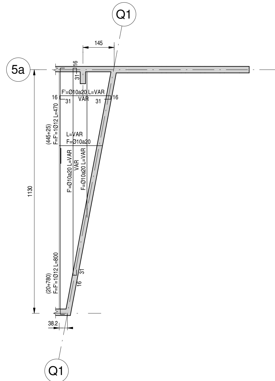
PLANTA ARMADURA DE LOSA NIVEL -0.02 ACCESO RAMPA PEATONAL ESCALA 1 : 100
