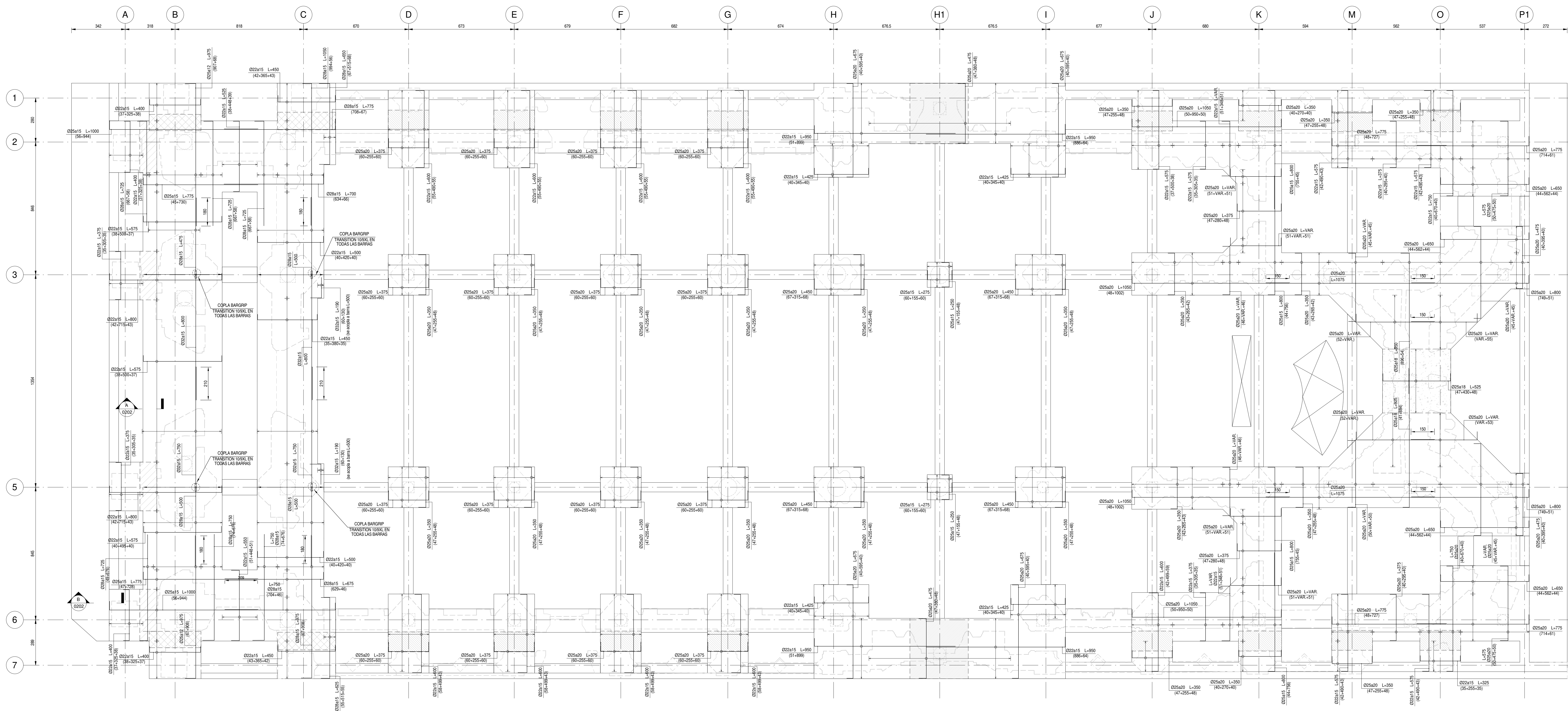
ETAPAS DE HORMIGONADO SEGUN DEFINIDO EN PLANO 103 Y CORTES PLANTA ARMADURA INFERIOR Y DE CORTE DE LOSA CIELO 1° SUBTERRANEO - 1° ETAPA ESCALA 1 : 100
