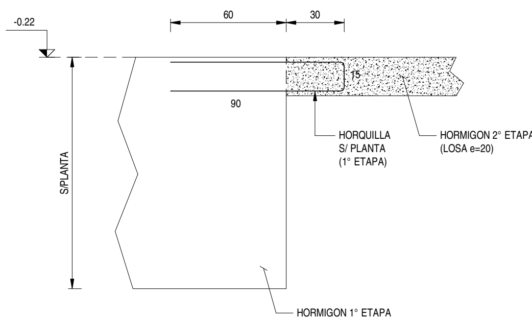
CORTE A ESC. 1 : 20
