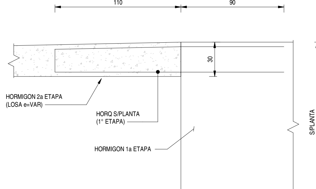
CORTE B ESC. 1 : 20
