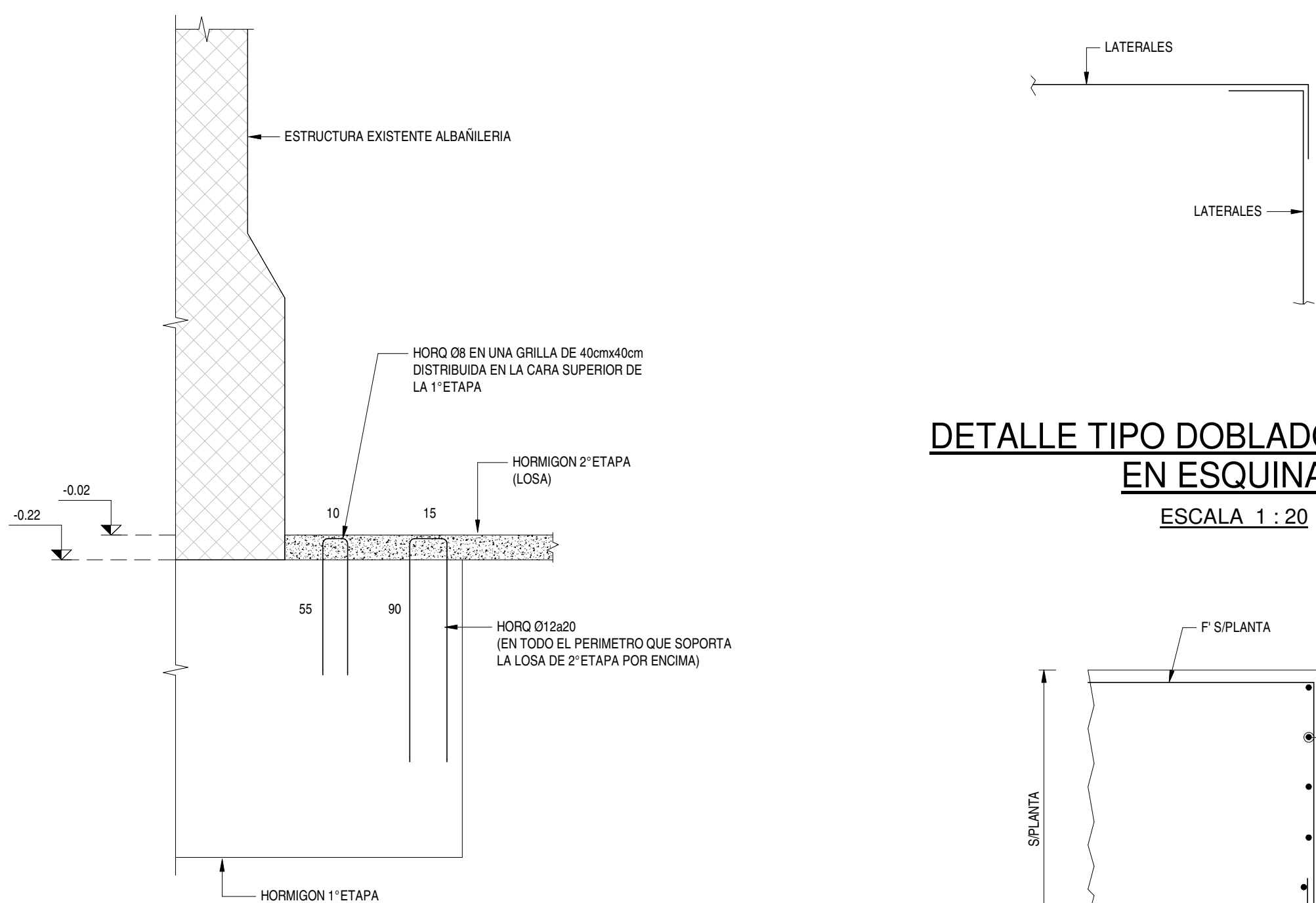
DETALLE TIPO HORQUILLAS DE UNION DE LOSA DE 2ª ETAPA COLOCADA SOBRE HORMIGON DE 1ª ETAPA ESCALA 1 : 20
