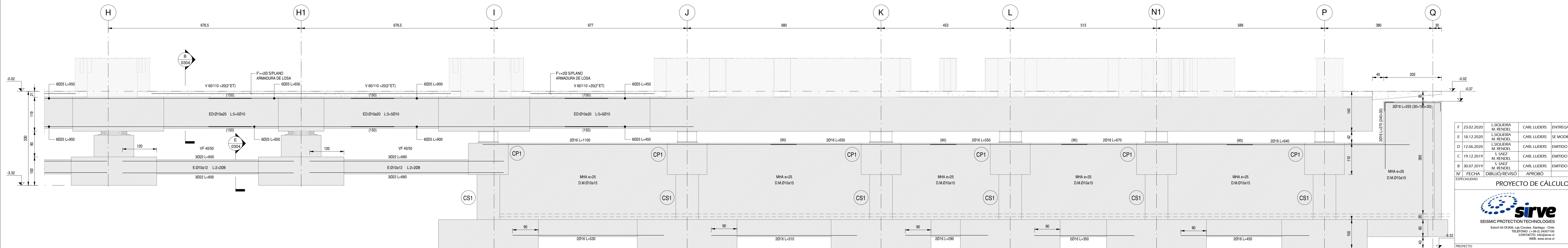
ELEVACION EJE 5 - ENTRE EJES H y P ESCALA 1 : 50
