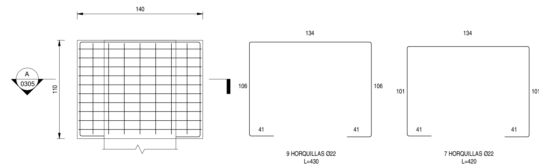
ARMADURA CAPITEL CP1 ESCALA 1 : 25
