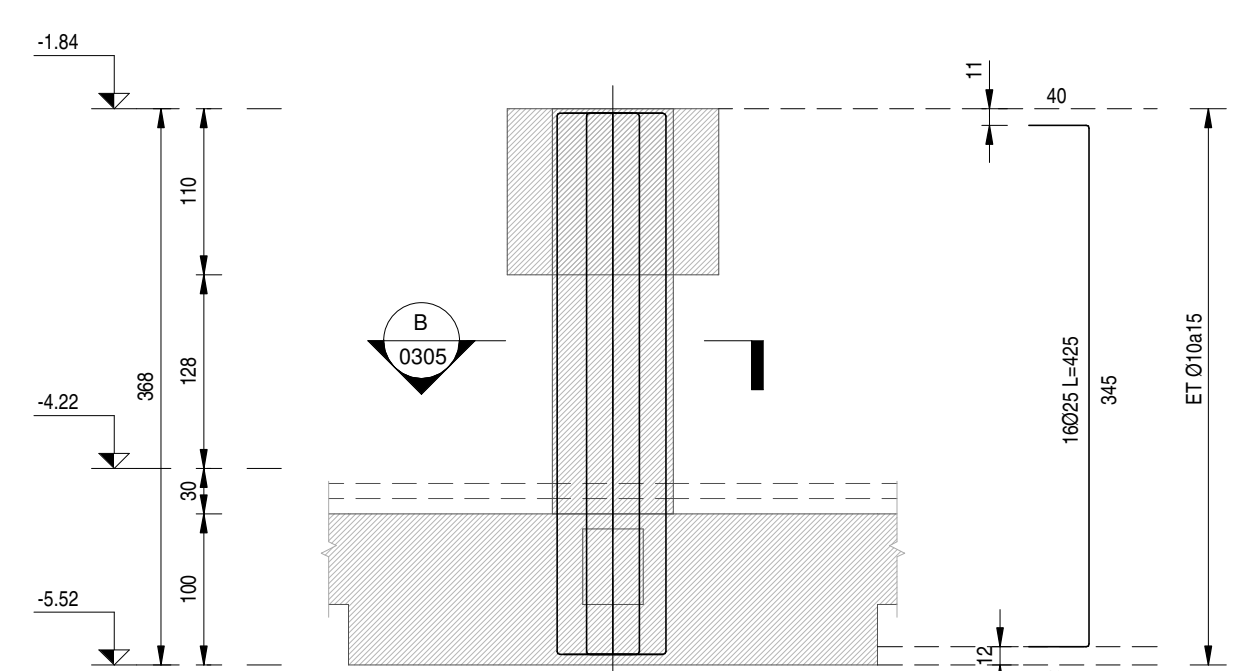
ELEVACION COLUMNA CS1 ESCALA 1 : 50
