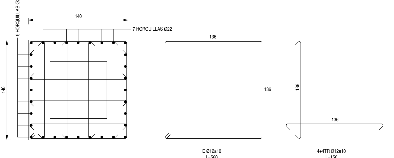
CORTE A ESC. 1 : 25
