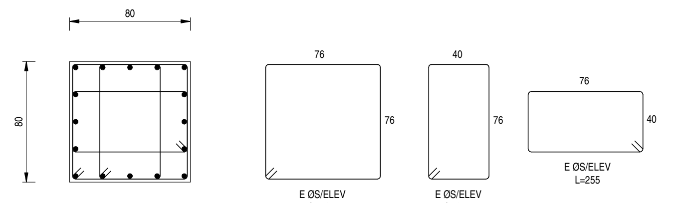
CORTE B ESC. 1 : 25
