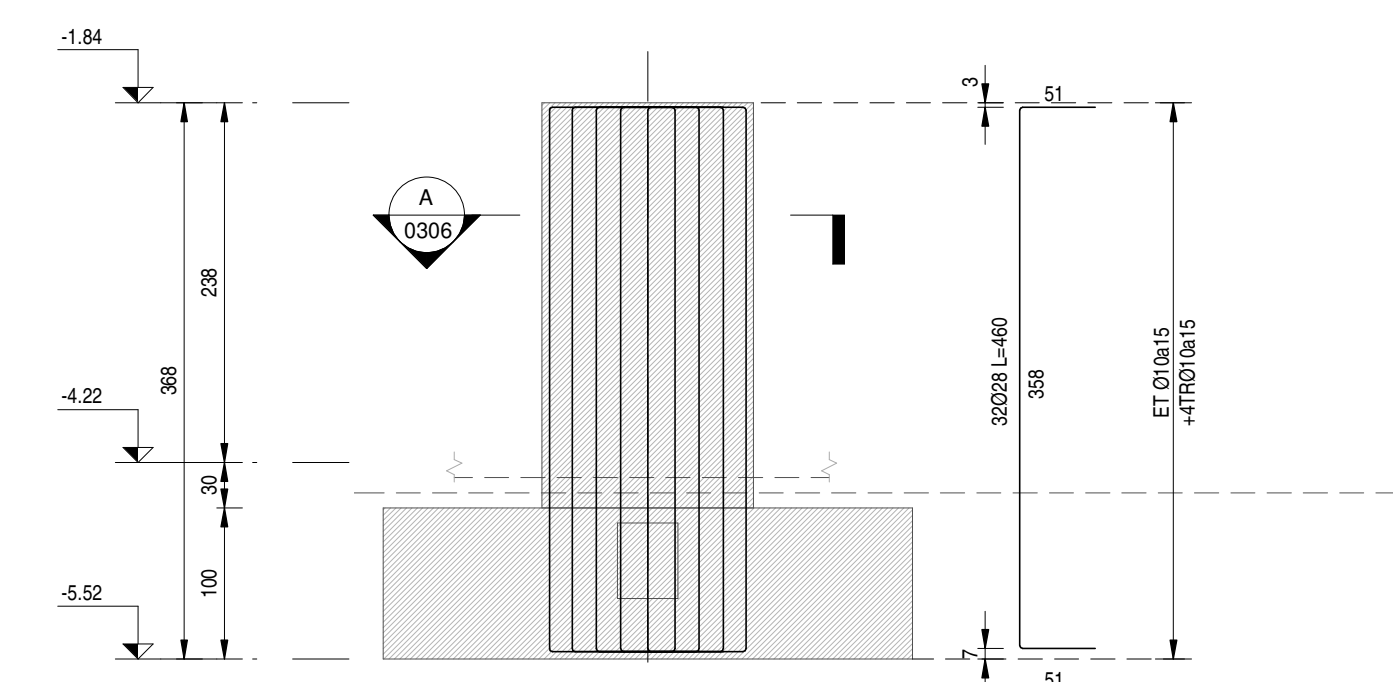
ELEVACION COLUMNA CS2 ESCALA 1 : 50
