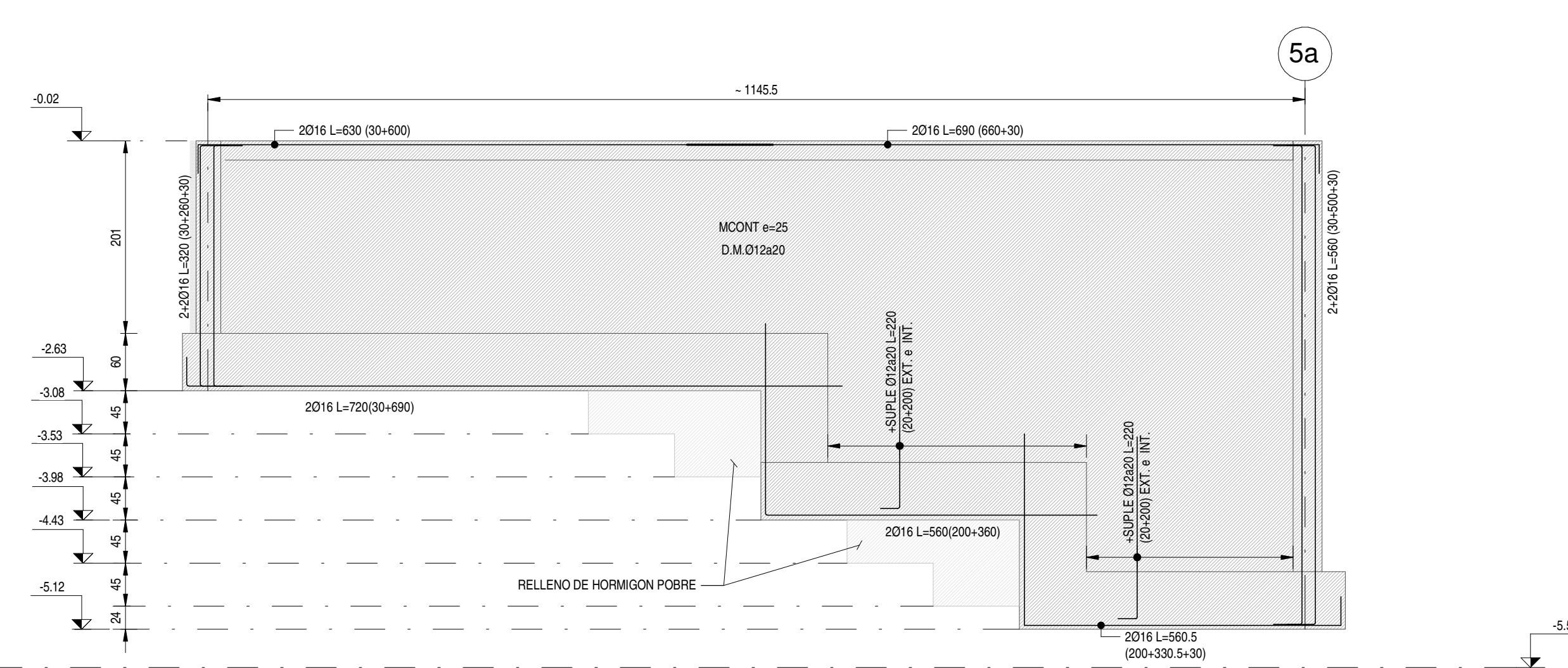
ELEVACION EJE Q1 ESCALA 1 : 50
