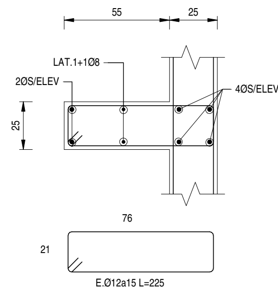
CORTE A ESC. 1 : 20
