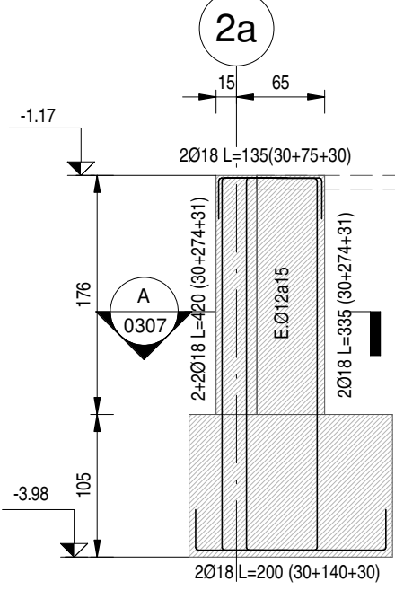
ELEVACION CONTRAFUERTE CF3 ESCALA 1 : 50
