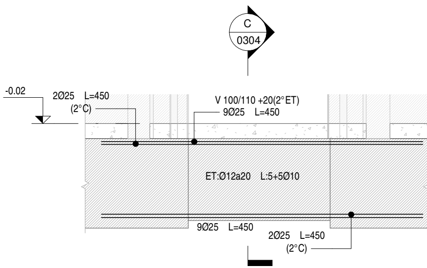
ELEVACION V102 ESCALA 1 : 50
