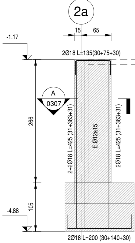
ELEVACION CONTRAFUERTE CF2 ESCALA 1 : 50
