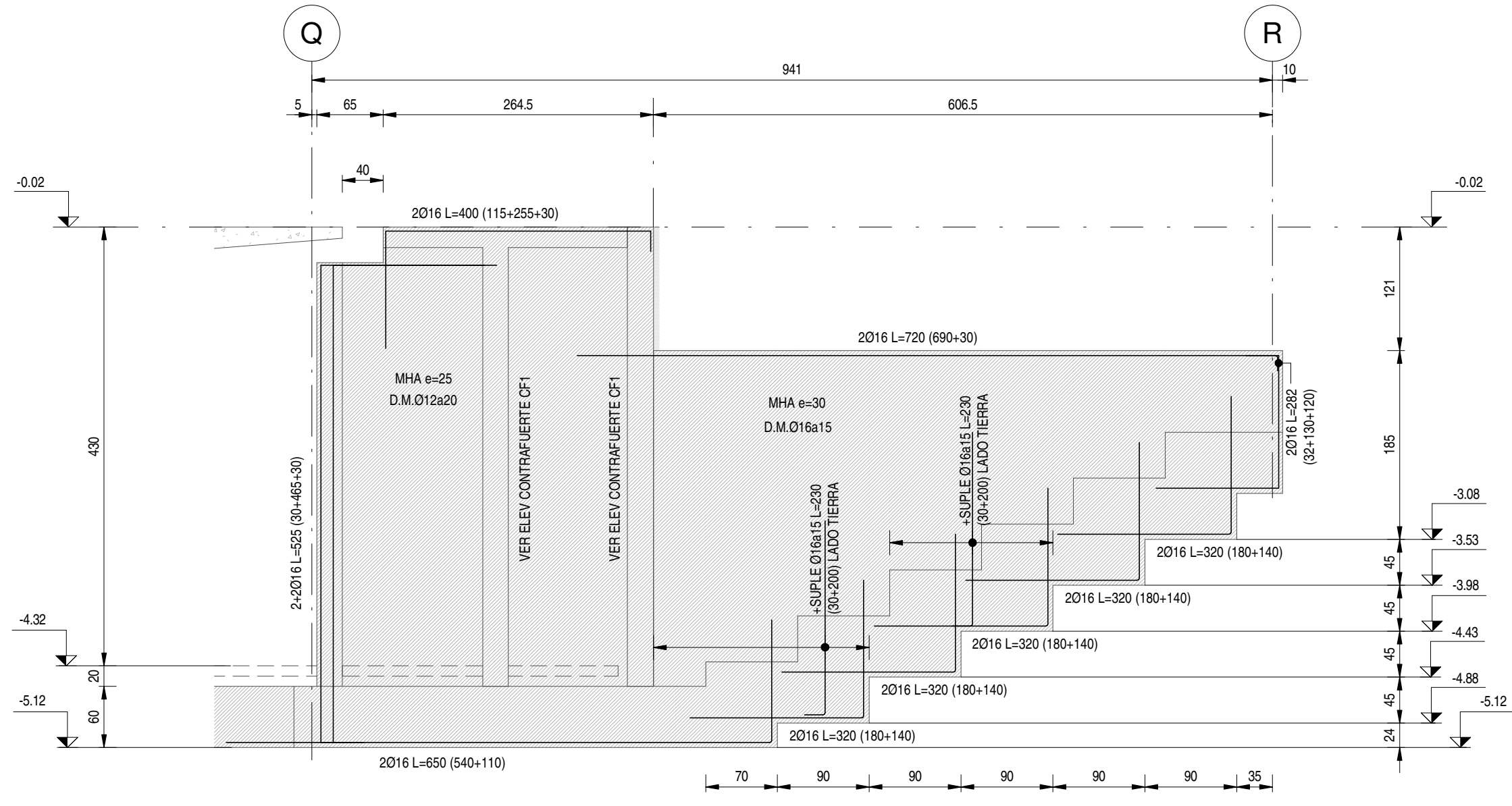
ELEVACION EJE 5a ESCALA 1 : 50
