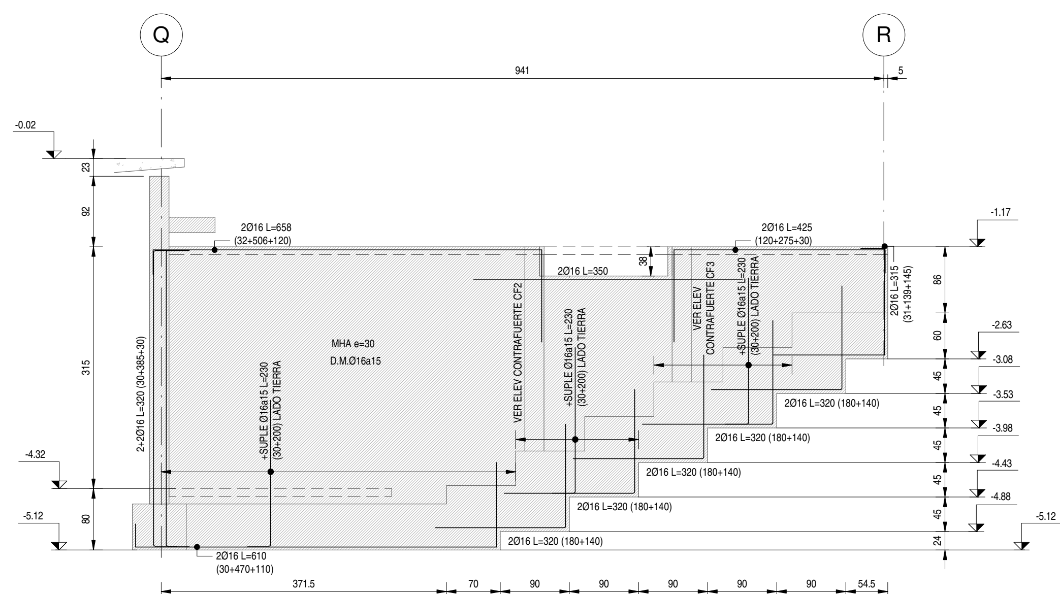
ELEVACION EJE 2a ESCALA 1 : 50
