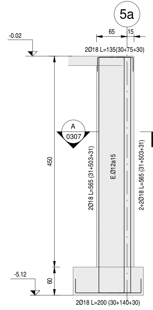
ELEVACION CONTRAFUERTE CF1 ESCALA 1 : 50
