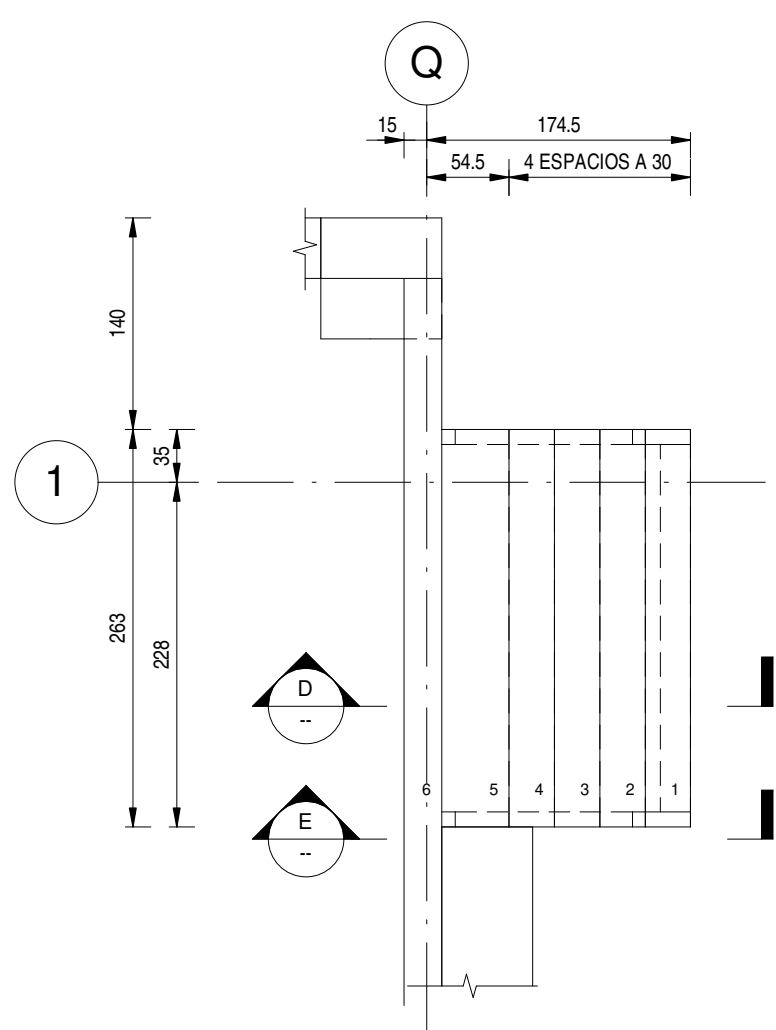
ESCALERA 2 PLANTA DE ESTRUCTURA ESCALA 1 : 50
