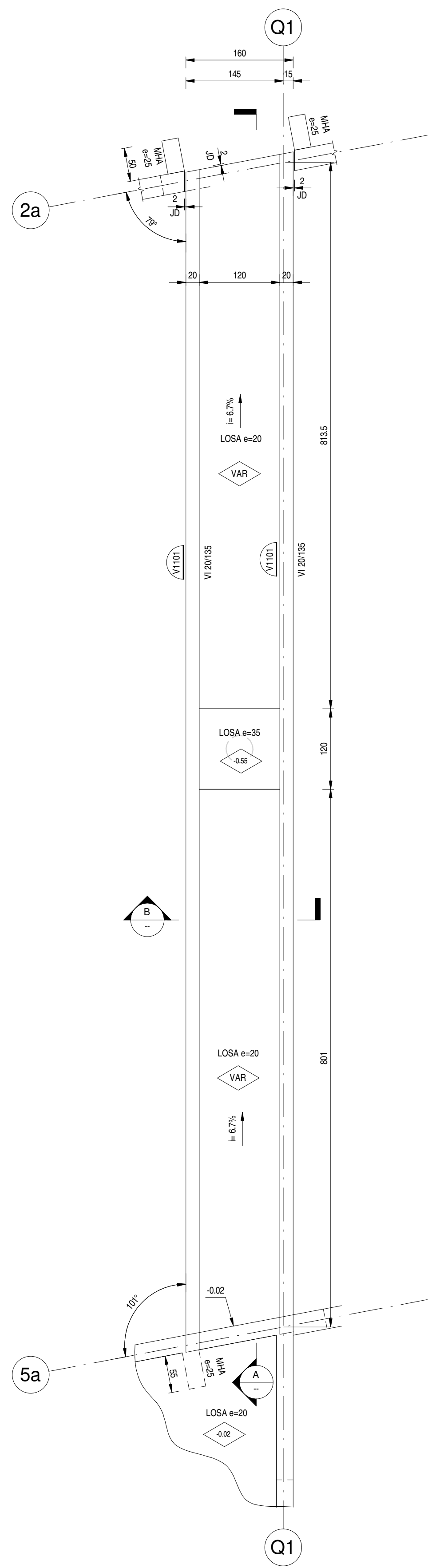
RAMPA PLANTA DE ESTRUCTURA ESCALA 1 : 50
