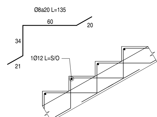
DETALLE DE GRADAS ESCALA 1 : 25
