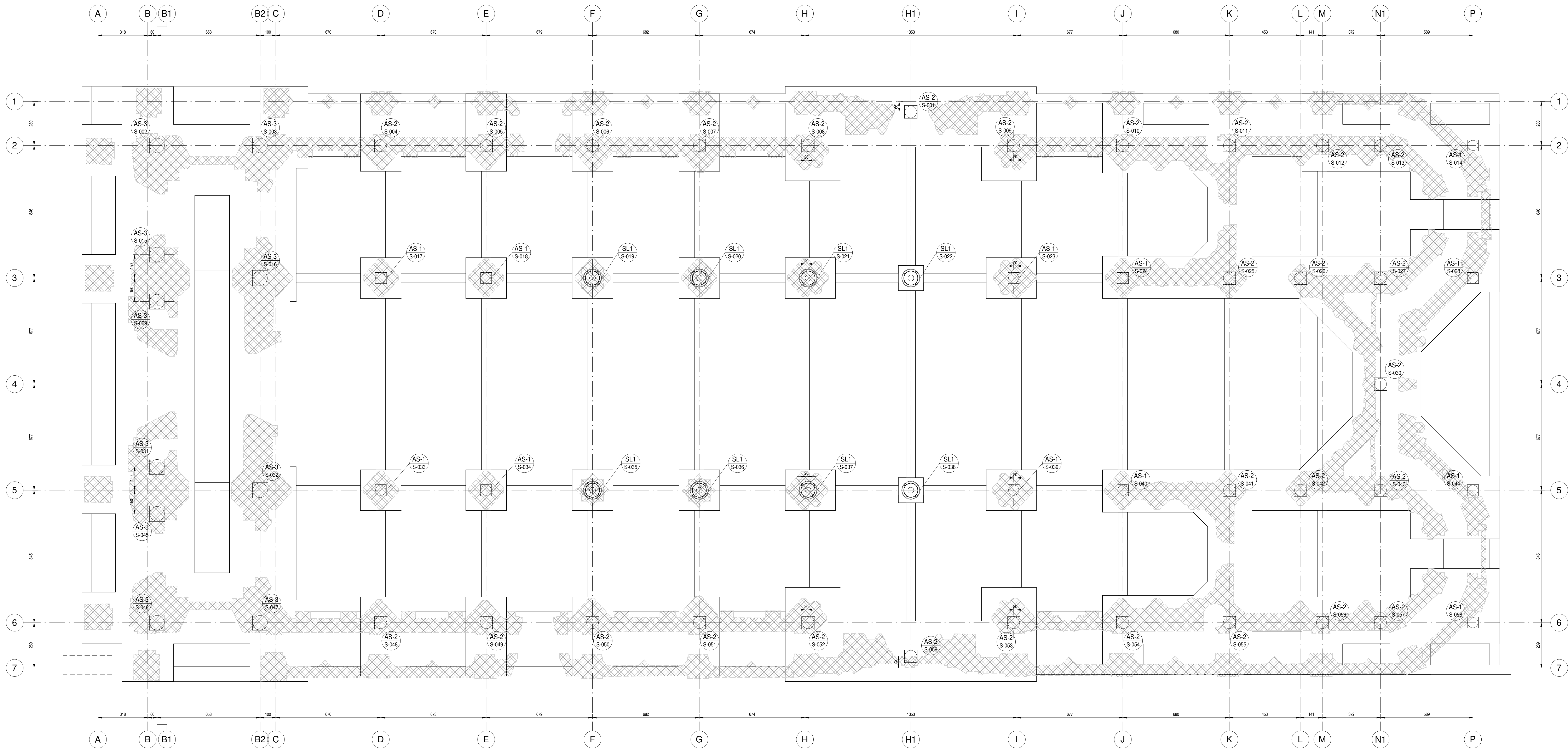
ELEMENTOS CENTRADOS A EJE (S.I.C.) PLANTA DE DISTRIBUCION DE DISPOSITIVOS ESCALA 1 : 100
