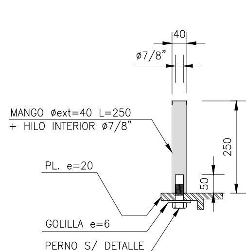
(DIMENSIONES EN mm.) DETALLE EMPALME PERNO Ø7/8" EN MANGO ESCALA 1:10
