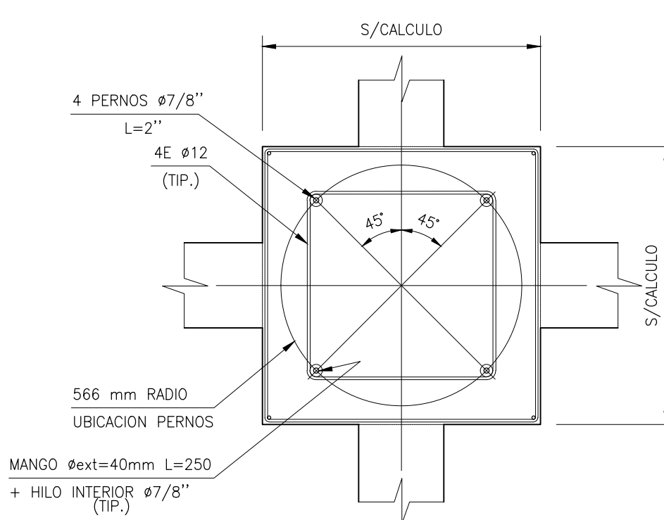
(DIMENSIONES EN mm.) CORTE B ESCALA 1:25
