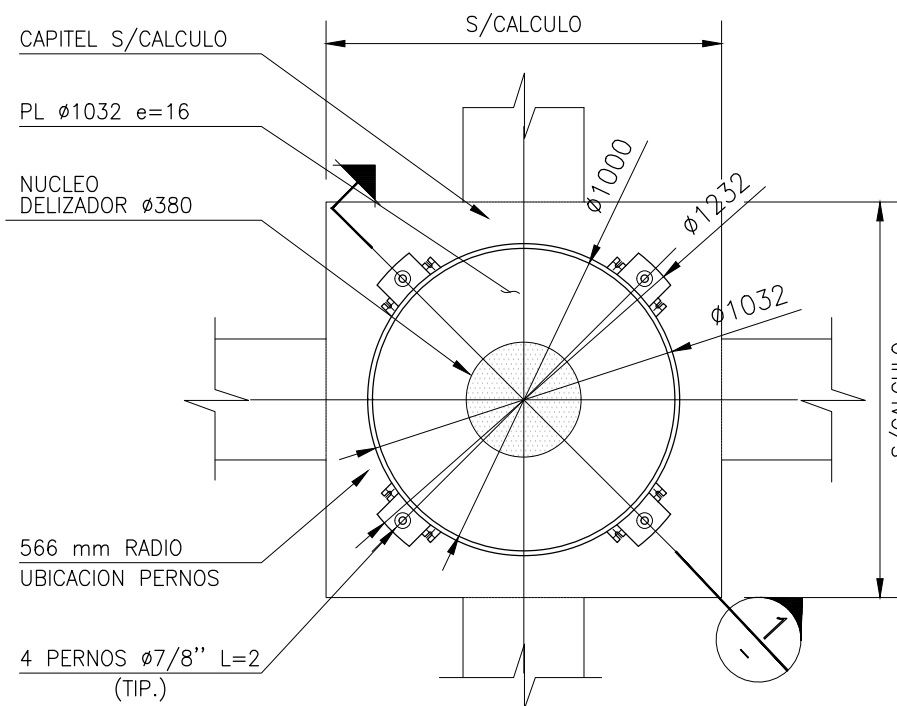
(DIMENSIONES EN mm.) CORTE A ESCALA 1:25
