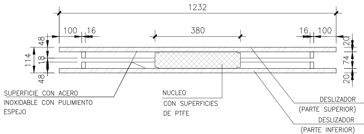
(DIMENSIONES EN mm.) SECCION DESLIZADOR (SL1) CORTE 1 ESCALA 1:10
