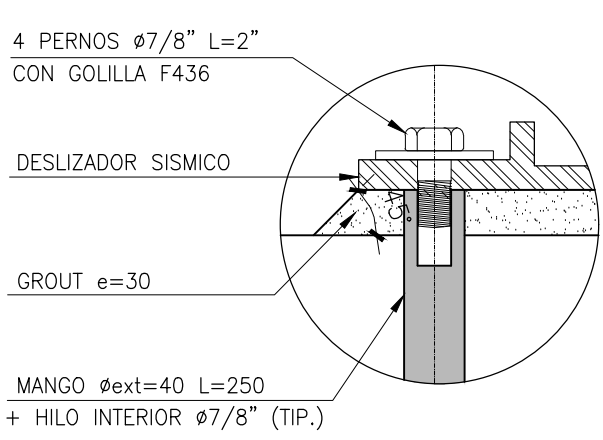
DETALLE 1 ESCALA 1:5
