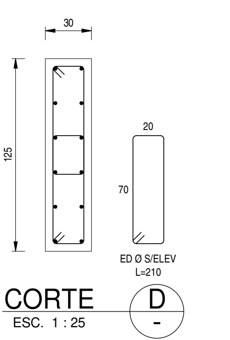
CORTE TIPOICO PILA P4
