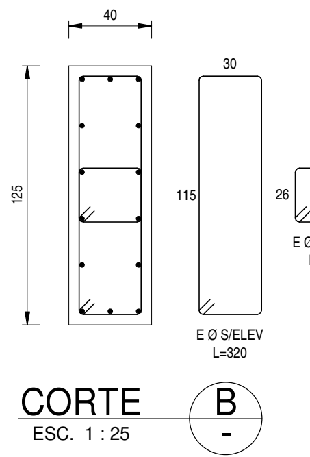
CORTE TIPOICO PILA P2
