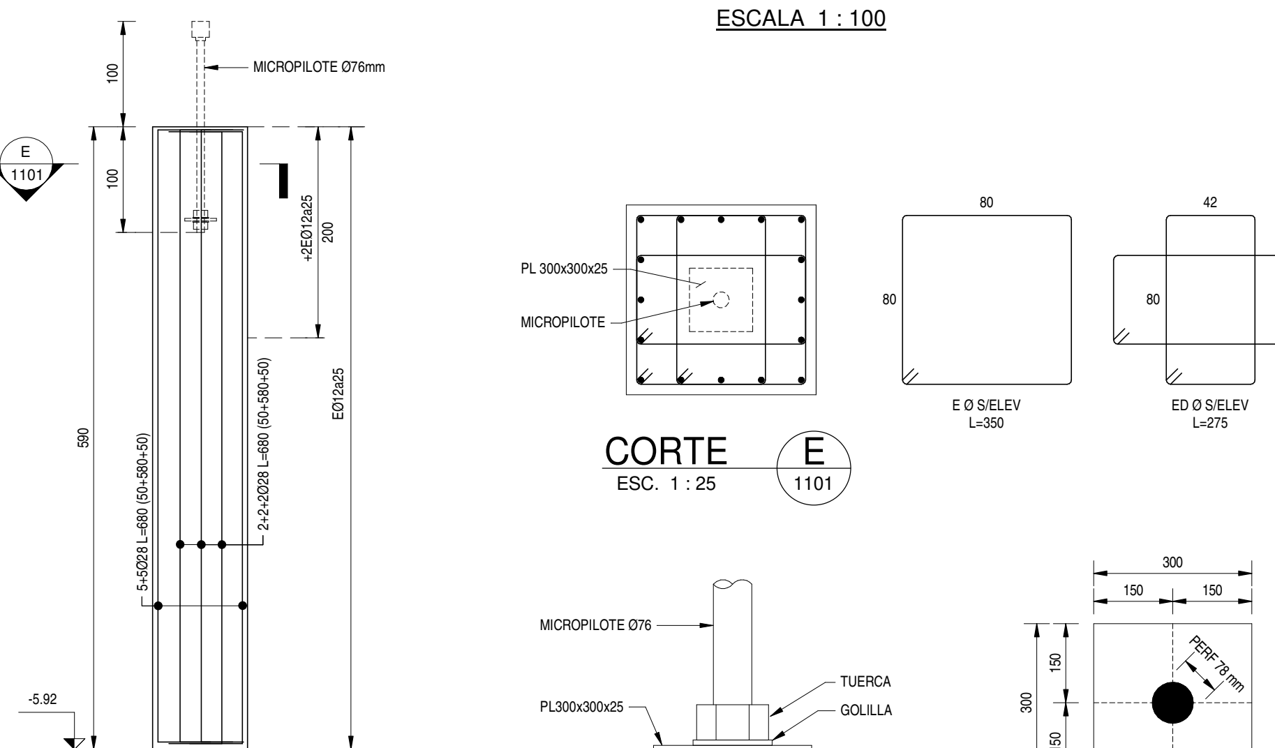
DETALLE TIPO DE PILA TEMPORAL DE HA
