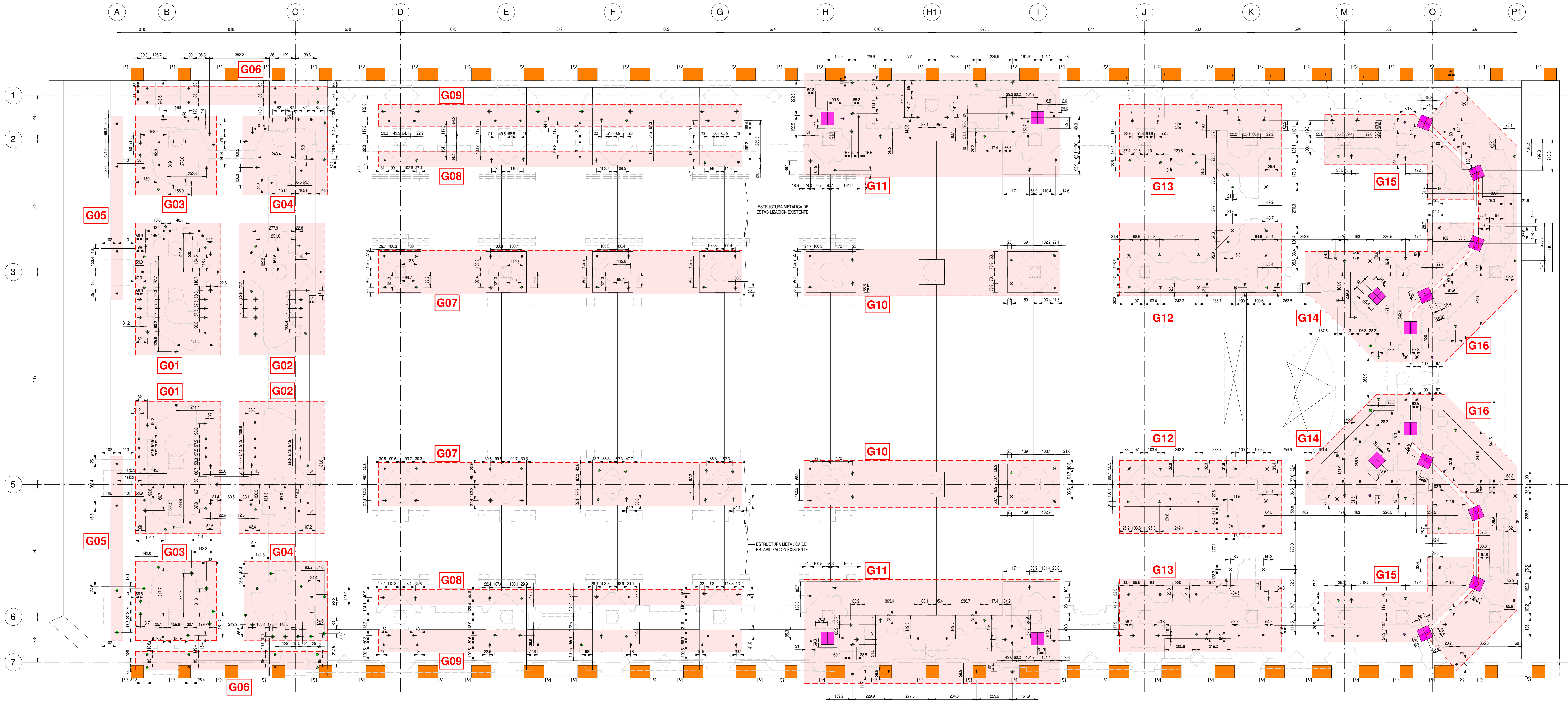
PLANTA DE DISPOSICION DE MICROPILOTES Y GRUPOS DE MICROPILOTES
