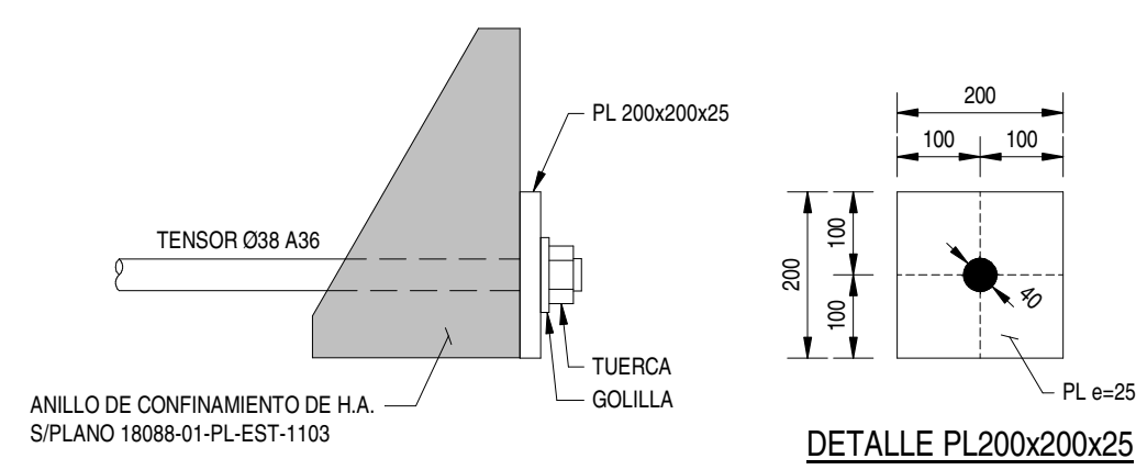
DETALLE TIPO DE TENSORES TERMINADOS EN PLACA ESCALA 1 : 10
