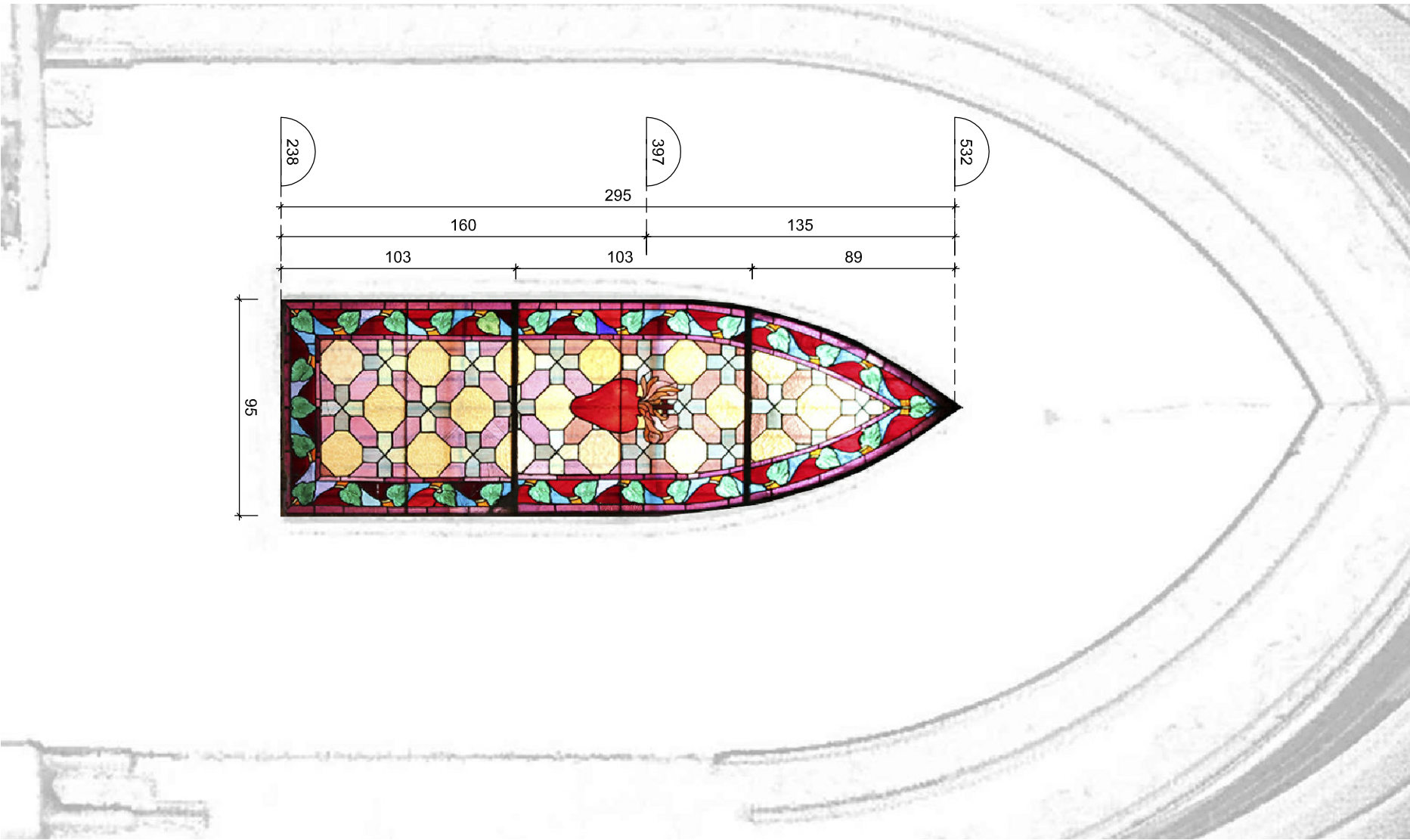
Elevación - Esc. 1/25
