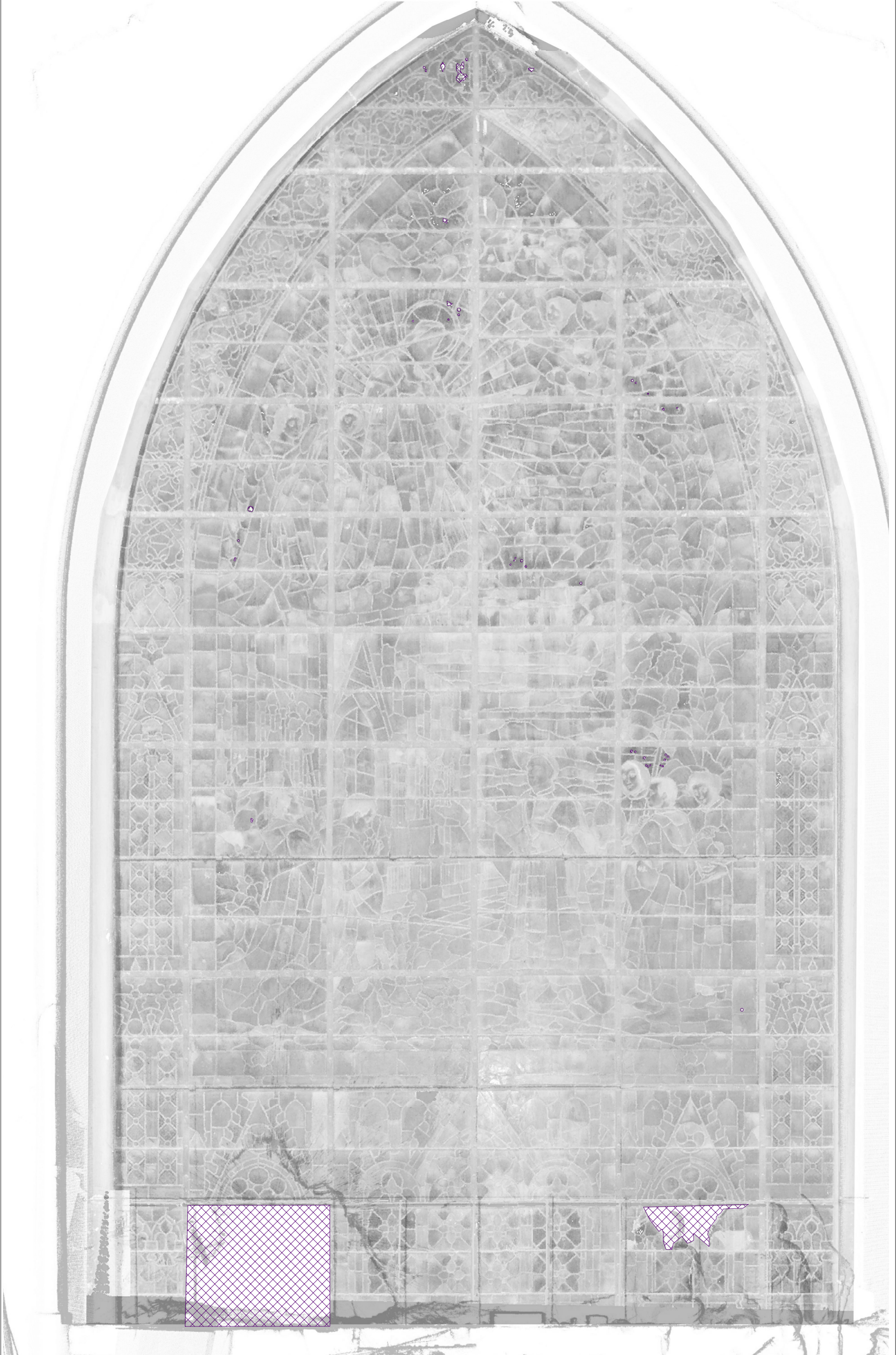
Levantamiento de daños. Esc. 1/25
