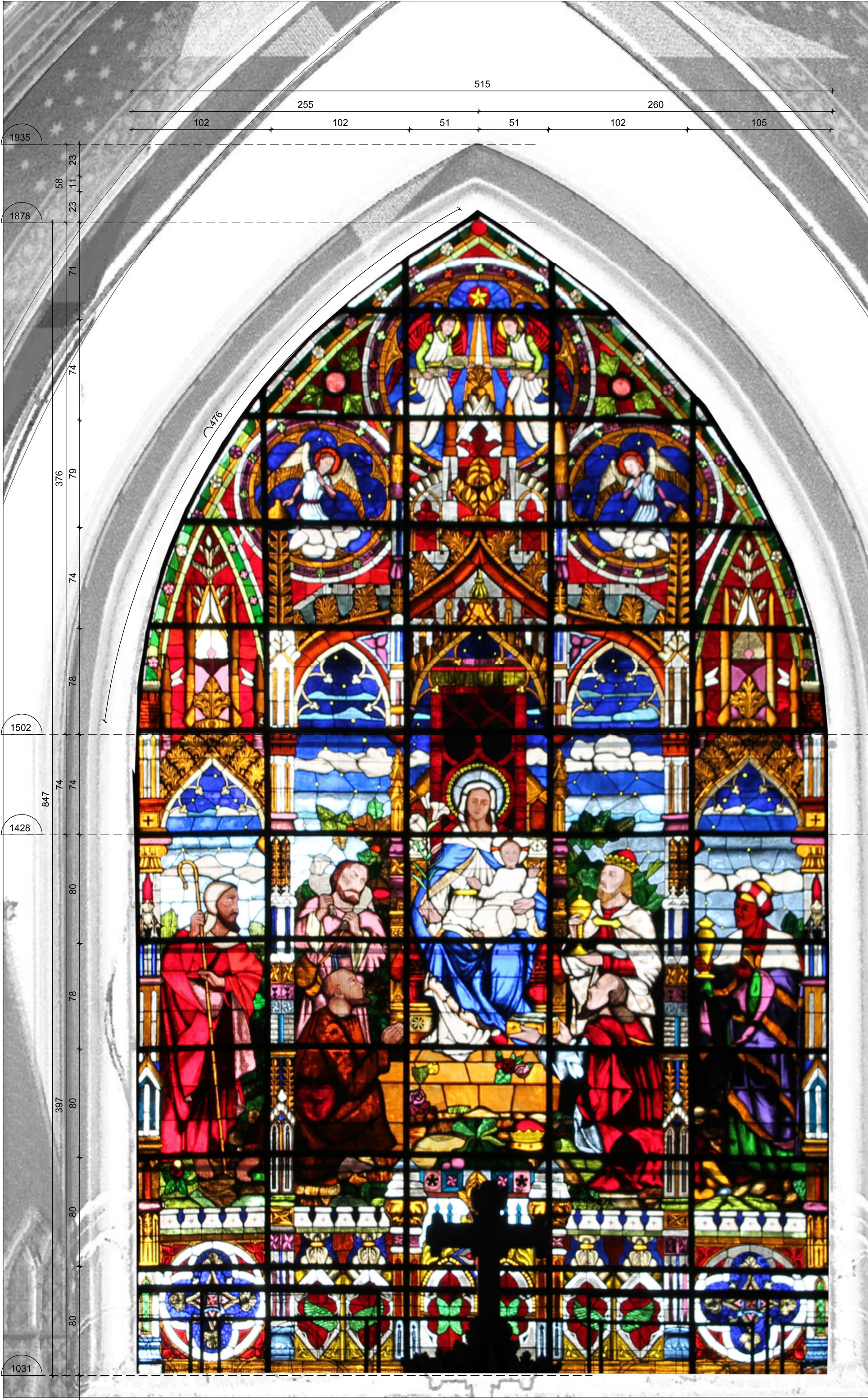
Elevación Esc. 1/25
