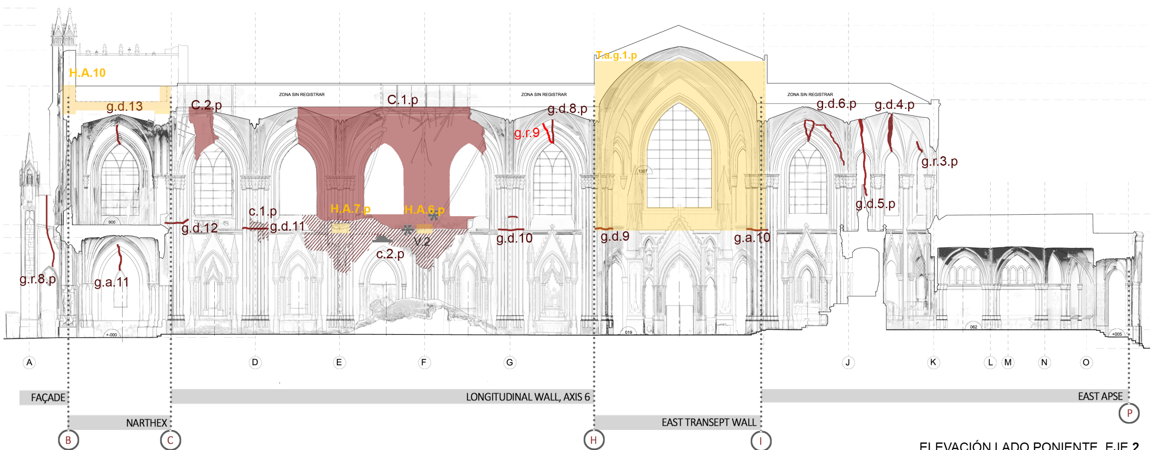
ELEVACIÓN LADO PONIENTE, EJE 2
