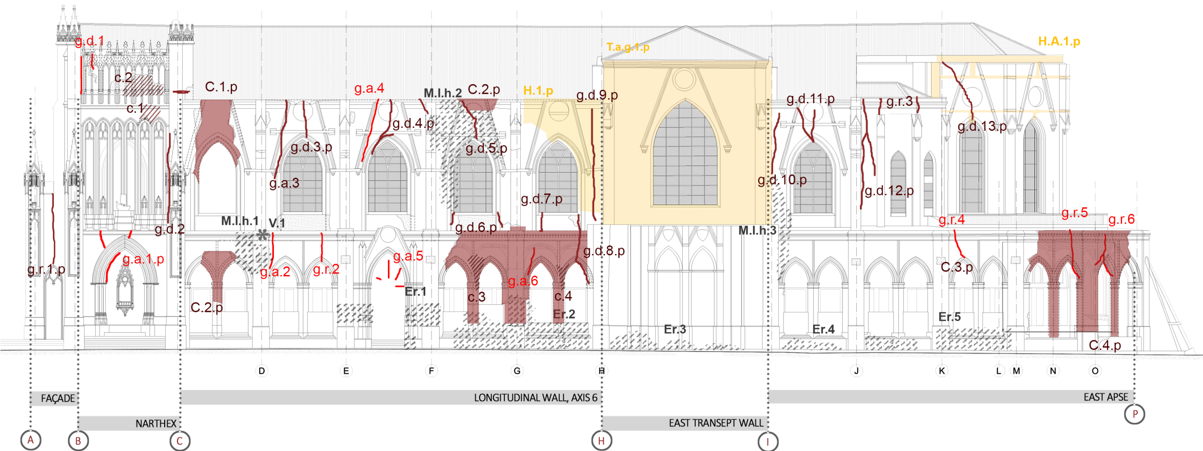
ELEVACIÓN LADO PONIENTE, EJE 6
