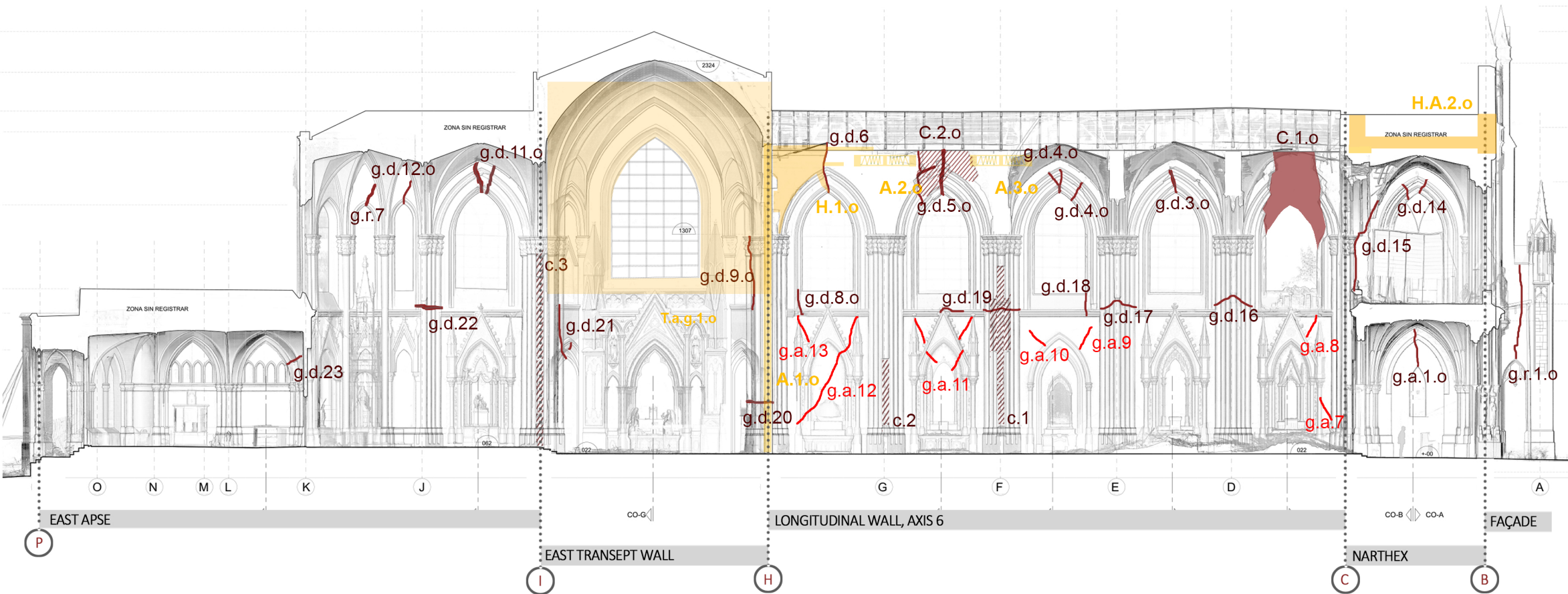
ELEVACIÓN LADO ORIENTE, EJE 6
